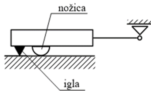
Slika 16. Prikaz vođenja igle ticala pomoću nožice [2]
