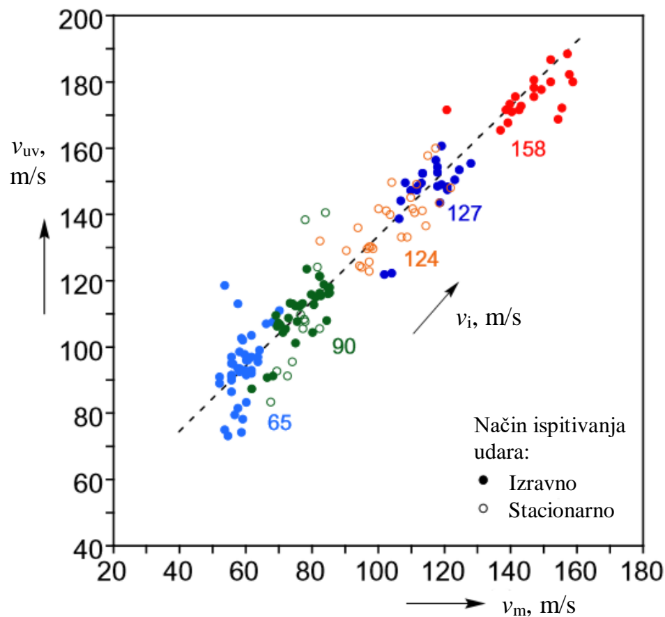
Slika 12. Odnos između brzine ispaljene mase i brzine udarnog vala [7]
