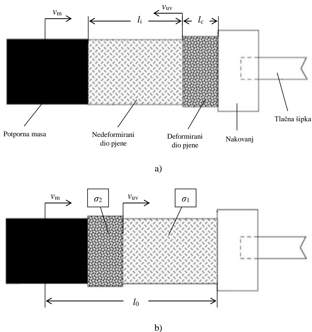
Slika 8. Dva načina ispitivanja udara s obzirom na početni položaj uzorka pjene: a) izravno b) stacionarno [7]
