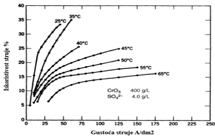
Slika 11. Iskoristivost struje u odnosu na gustoću struje [26]
