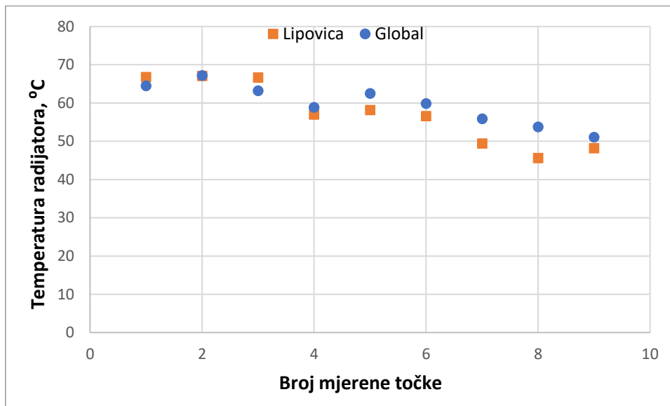
Slika 17. Temperature površine radijatora za režim 75/65
