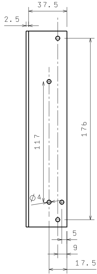
Bokocrt Mjerilo: 1:2
