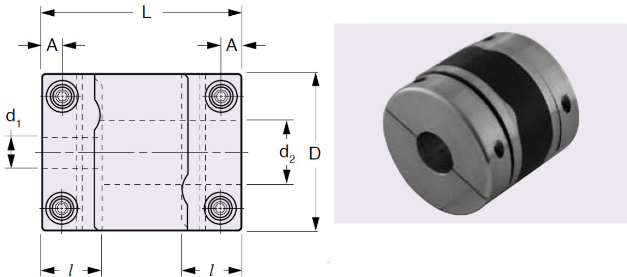
Slika 3.10 Spojka
