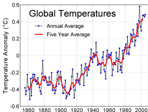
Slika 8.1 Temperaturne anomalije kroz posljednih 150 godina [5]
