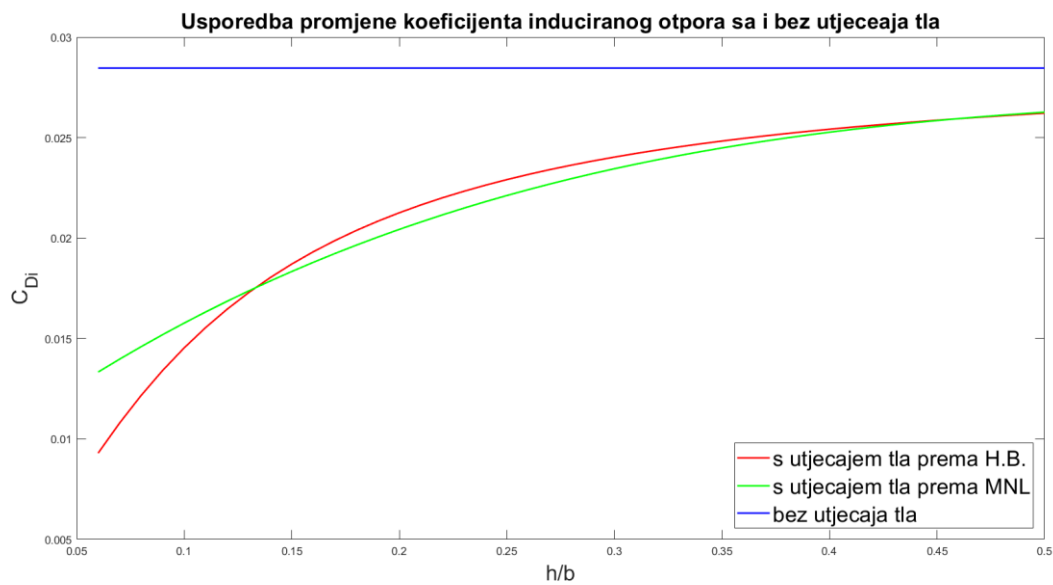
Slika 17 Usporedba promjene koeficijenta induciranoeg otpora u ovisnosti o h/b
