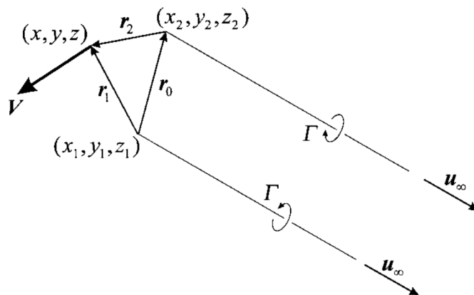
Slika 2.2: Brzina u točki (x, y, z) inducirana \Pi vrtlogom
