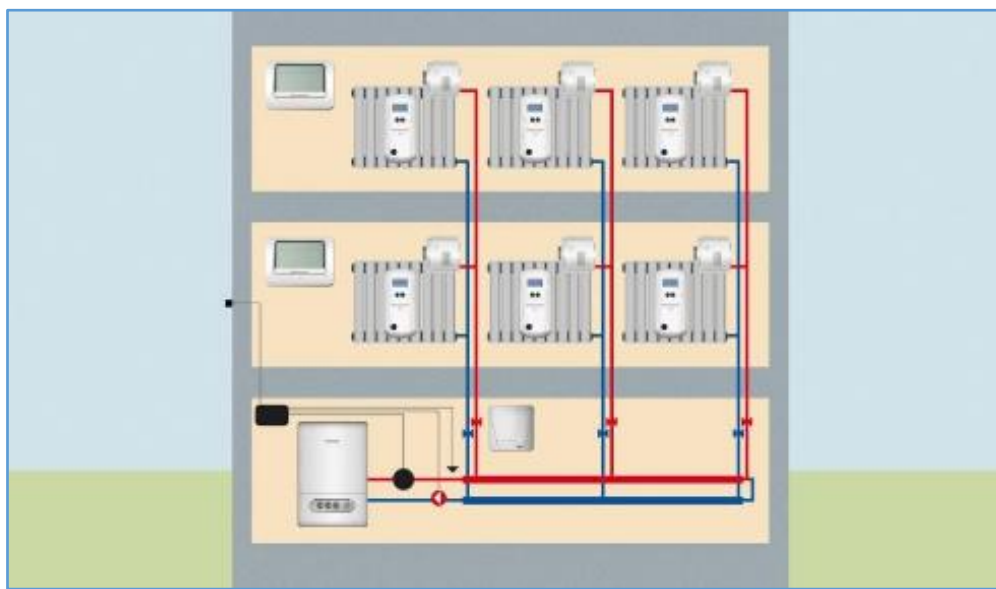
Slika 1-3 Shema ugradnje razdjelnika troškova toplinske energije unutar zgrade (Izvor: Honeywell)
