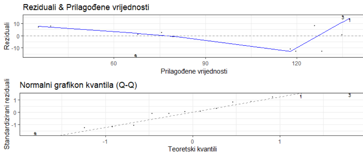
Slika 3-77 Dijagram reziduala i prilagođenih vrijednosti i normalni dijagram Q-Q za model na nacionalnoj razini
