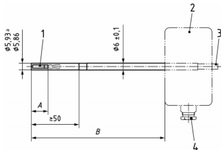
Slika 8. Tip PL temperaturnog senzora [4]
