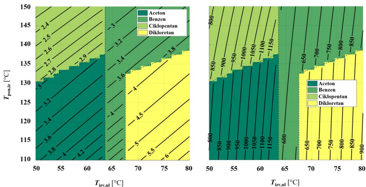
Slika 10. Najučinkovitije radne tvari iz priloga B s pripadajućim COP (lijevo) i q_{kond,v} vrijednostima (desno) [15]
