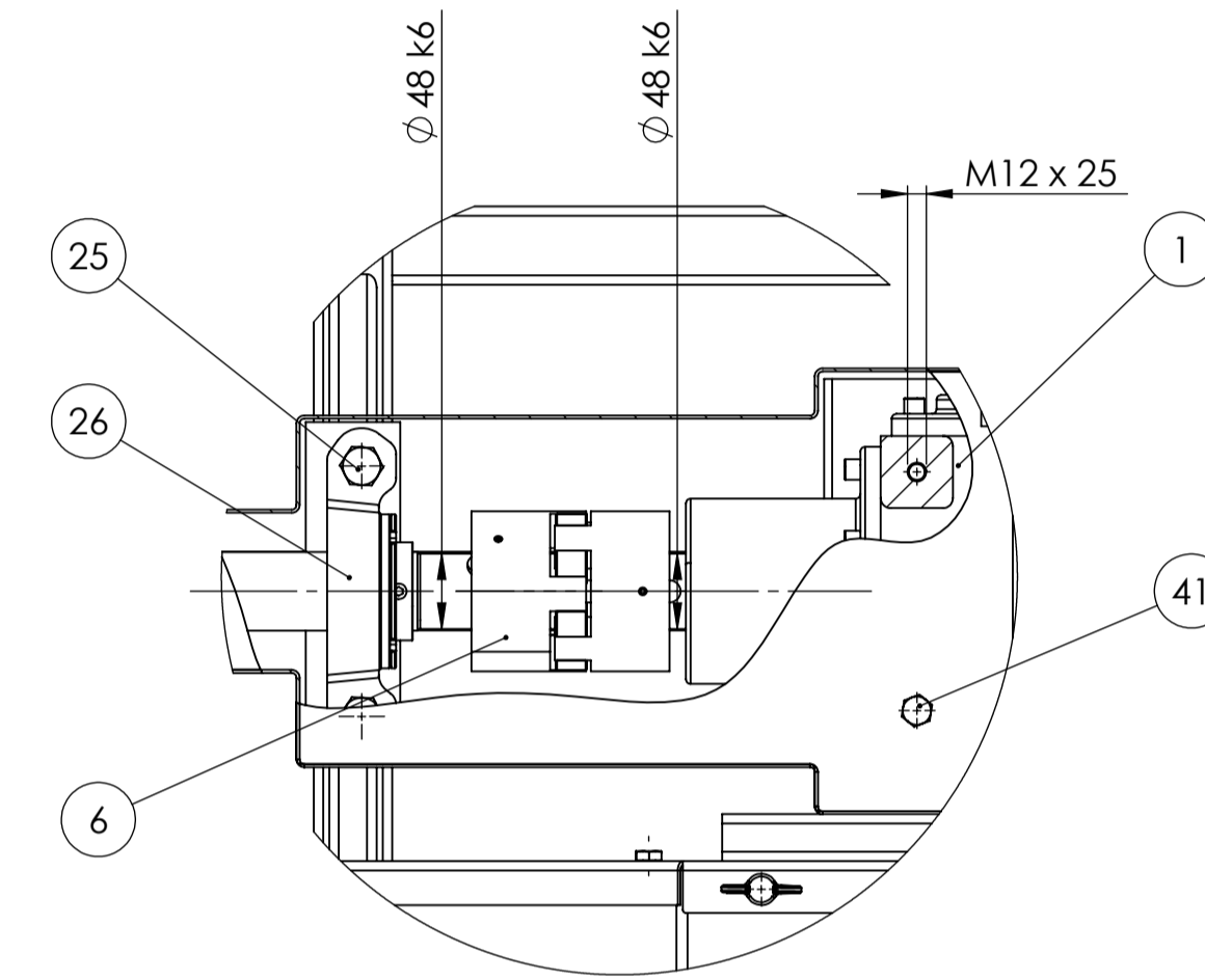
DETALJ T 1:5
