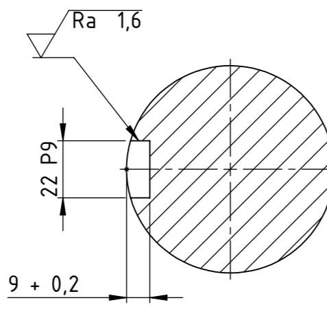
PRESJEK Z-Z 1:2
