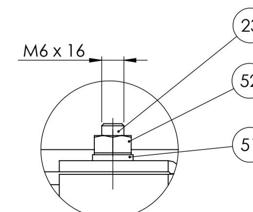
DETALJ N 1:1
