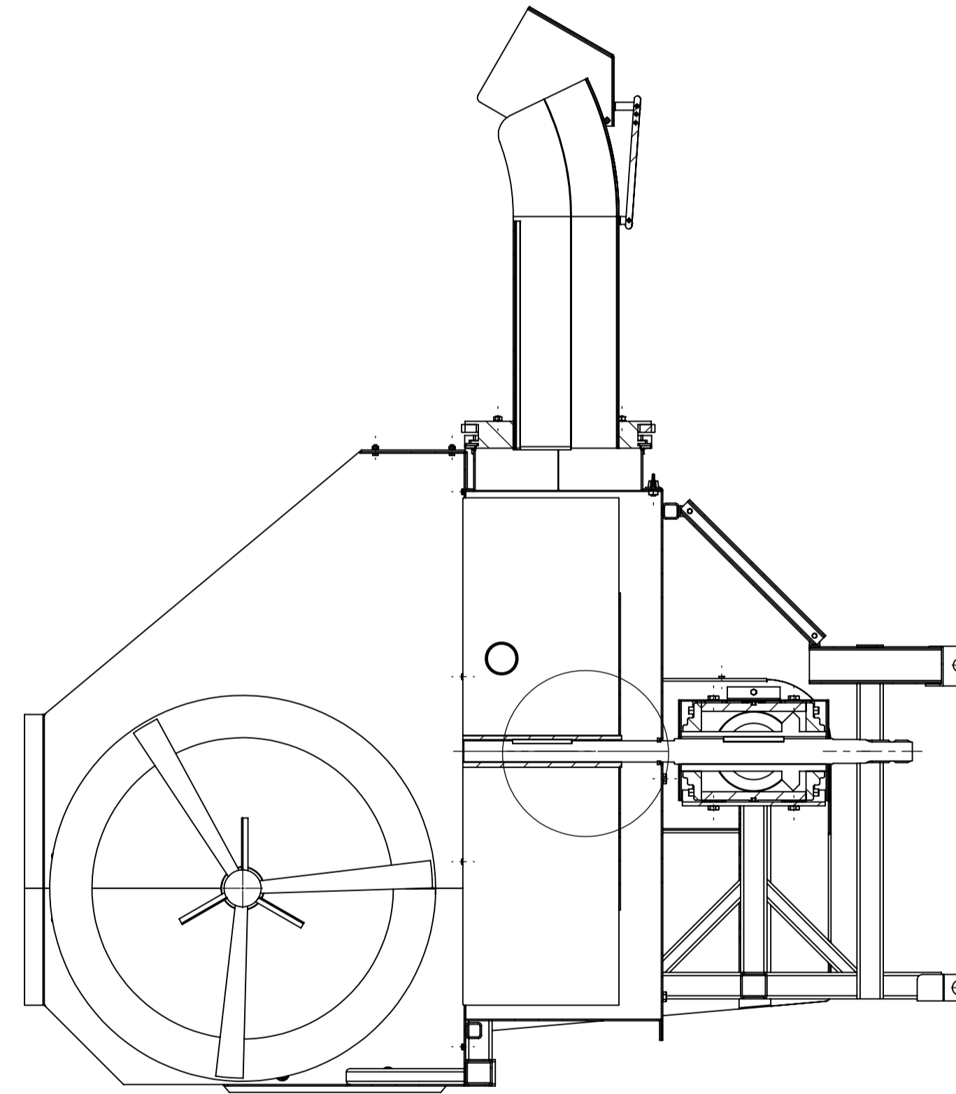
PRESJEK Q-Q
