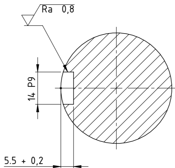
PRESJEK Y-Y 1 : 1
