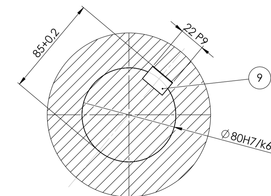
DETALJ R 1:2
