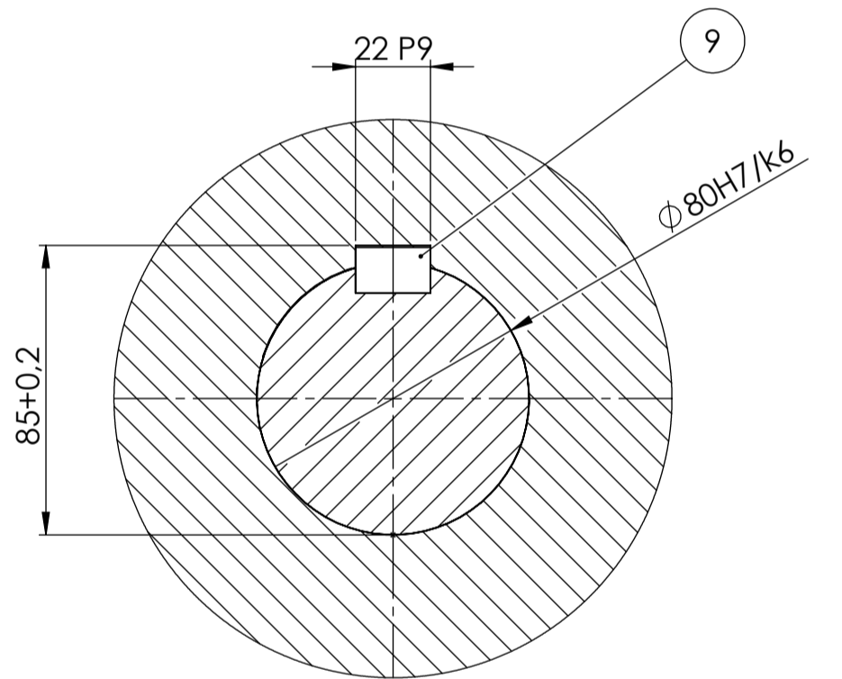
DETALJ S 1:2
