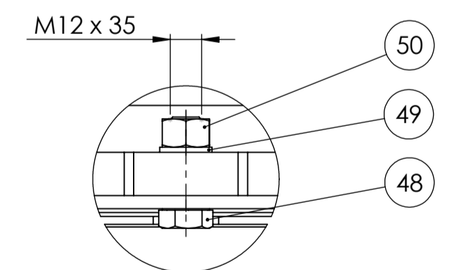
DETALJ P 1:2
