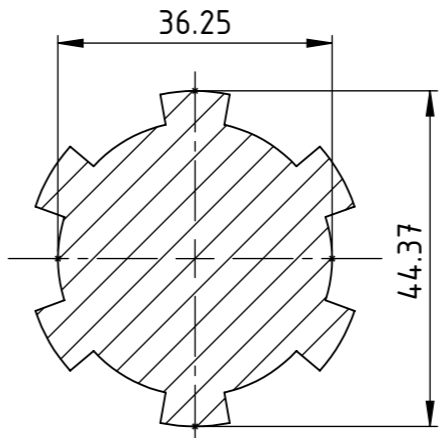
PRESJEK X-X 1 : 1
