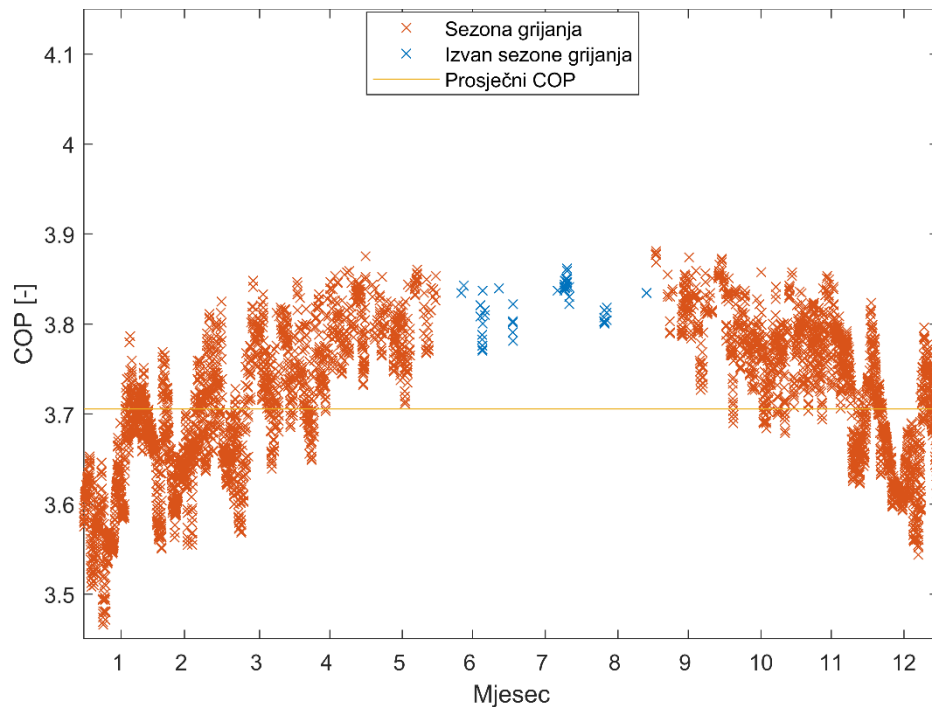
Slika 32: Faktori grijanja za svaki pojedini radni sat dizalice topline, „on/off“ način rada
