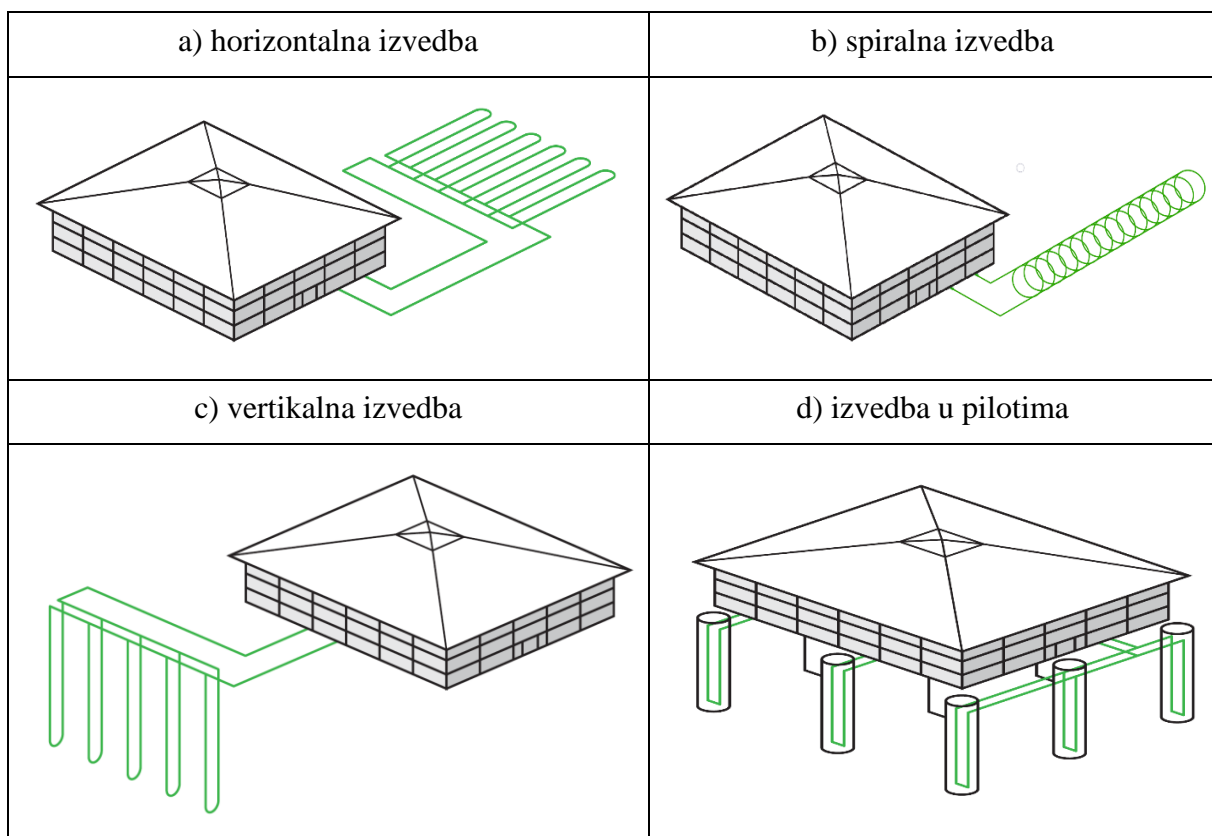
Slika 6: Vrste sekundarnih krugova zatvorenog indirektnog sustava geotermalne dizalice topline, izvor [33]
