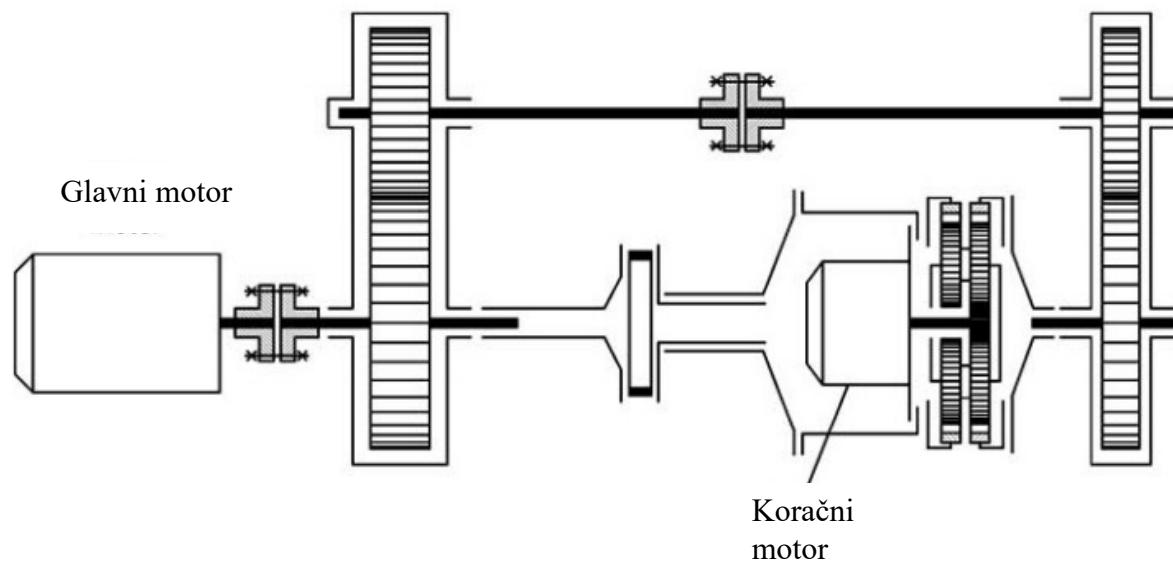
Slika 21. Ispitni uređaj sa Wolfromovim prijenosnikom [5]
