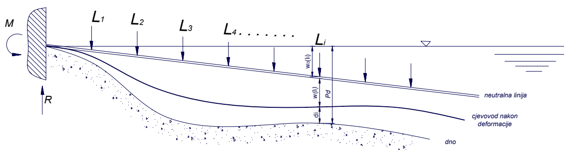
Slika 4.8 Sile od ovješnih lanaca
