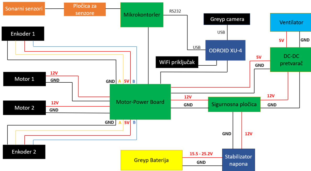
Slika 31. Električna shema spajanja komponenti mobilnog robota
