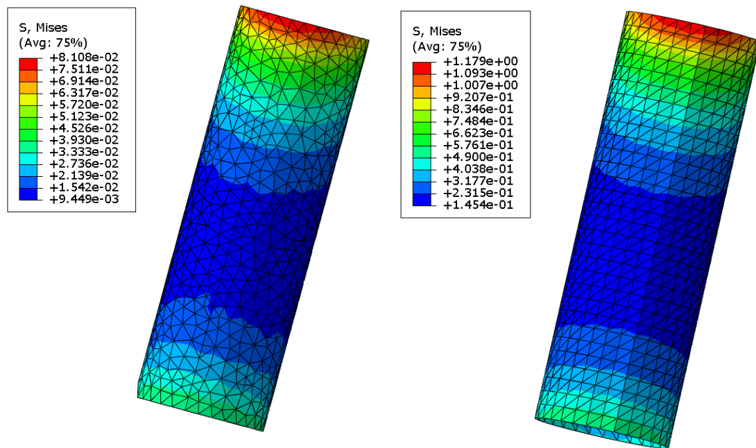
Slika 85. Naprezanja na unutarnjim modelima ljepila gornjeg sklopa, Skid pad
