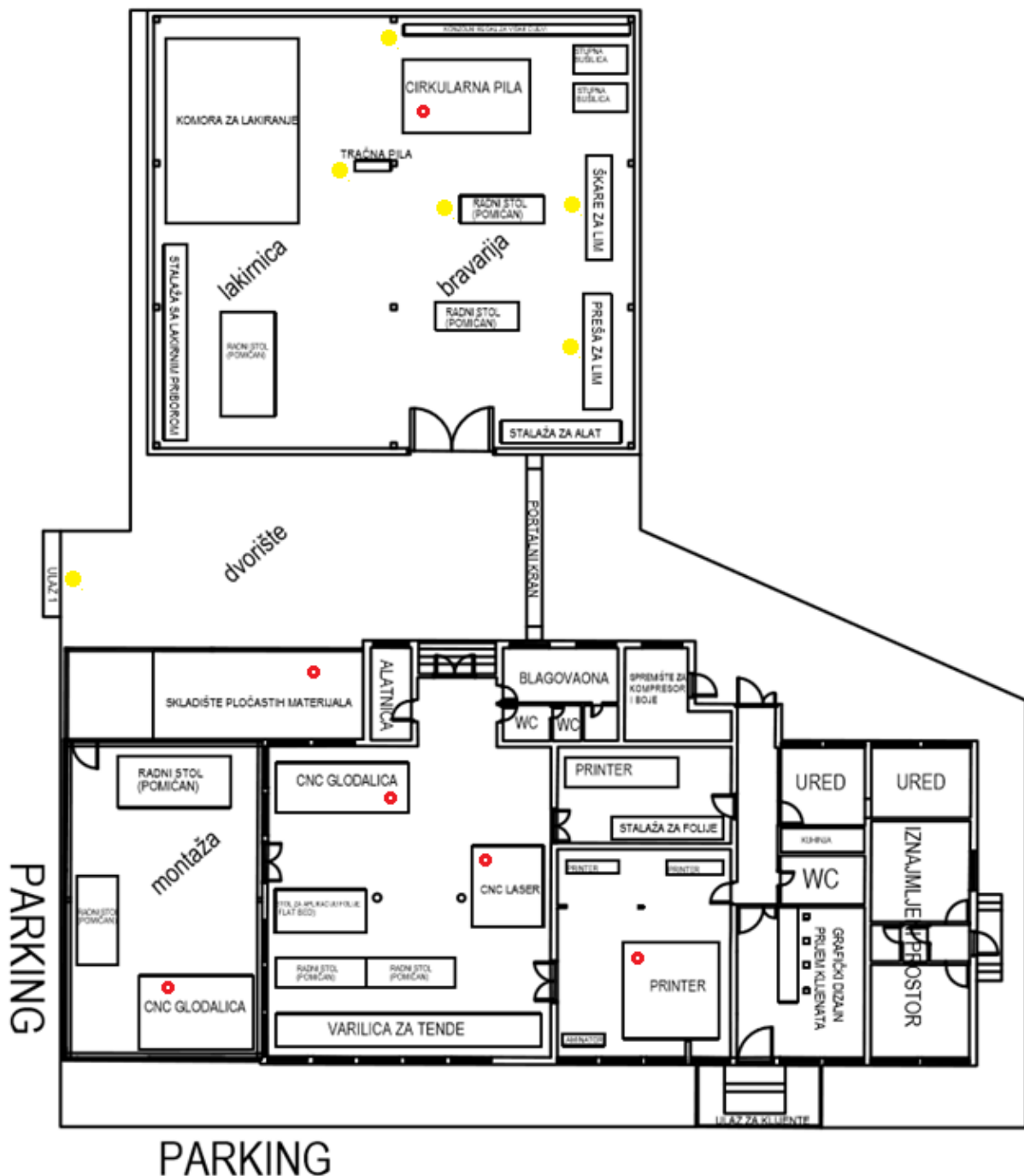
Slika 31. Tlocrt poduzeća
