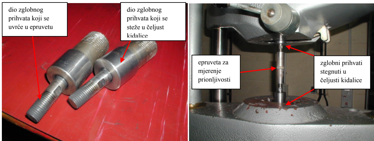
Slika 3.14 Zglobni prihvatni za eliminaciju momenta savijanja kod razvlačenja epruveta i njihov položaj u čeljustima kidalice.
