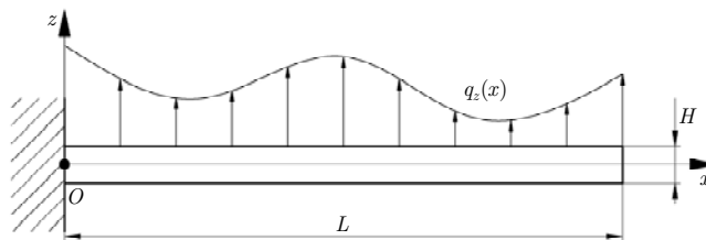
Slika 3.3 Poprečno ravno savijanje (jednostrano uklještena) monotone grede.
