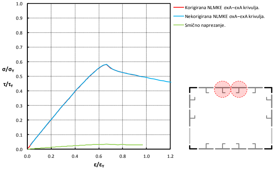
Slika 4.72 Uzdužna i smična nosivost diskretnih sastavnih elemenata („unutrašnjih“) ukrepa sa sunosivom širinom oplata gornjeg pojasa konstrukcije P1A pri R2.
