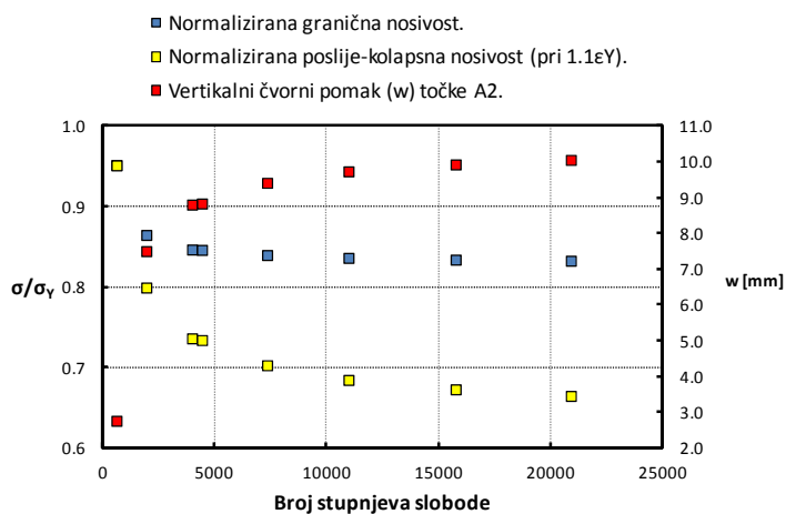
Slika 4.12 Usporedba rješenja dobivenih za različite rezolucije mreže razmatranog modela (srednja razina /Pravila/ IGO).
