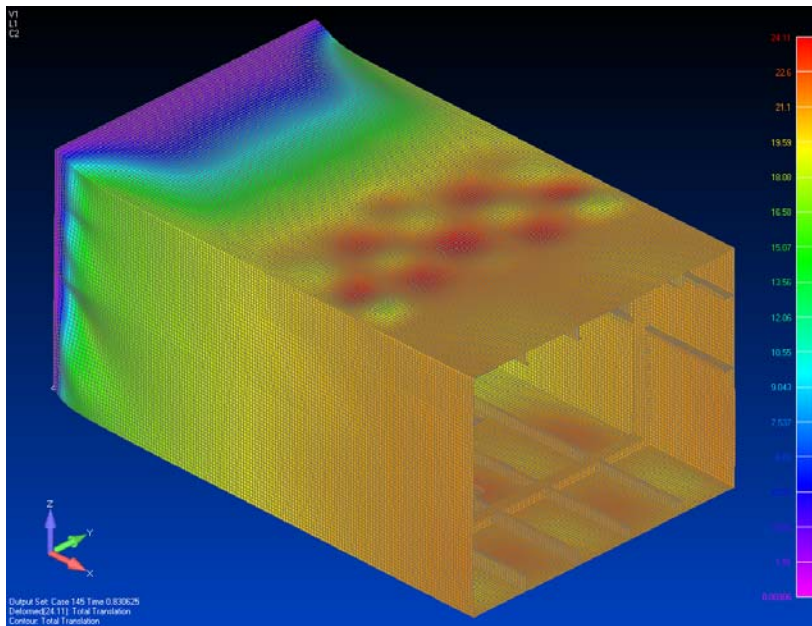
Slika 4.58 Deformirani NLME model konstrukcije P1A u graničnom stanju nosivosti (R1): Ukupni pomaci (karikirani) [mm].
