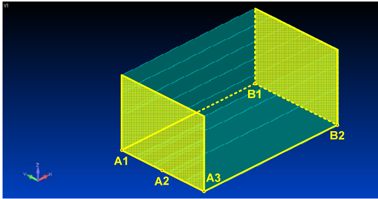
Slika 4.27 Mjesta zadavanja ograničenja popočenih pomaka i opterećenja za diskretizirani NLMKE model konstrukcije P1.
