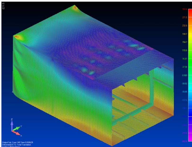
Slika 4.59 Deformirani NLME model konstrukcije P1A u graničnom stanju nosivosti (R1): \sigma_x za središnju plohu (eng. mid-plane ) elemenata [N/mm 2 ].
