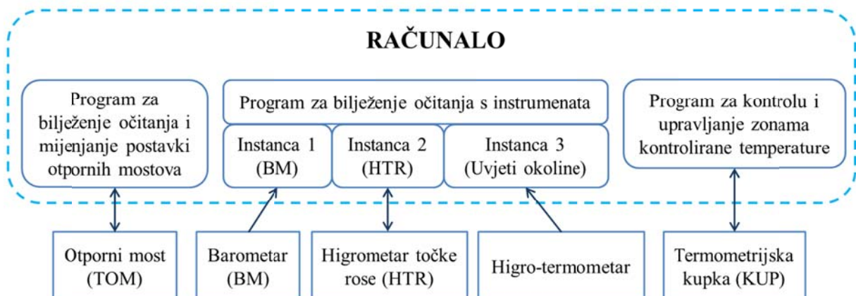
Slika 26. Shematski prikaz računalskih programa razvijenih za potrebe bilježenja očitavanja i upravljanje instrumentima.
