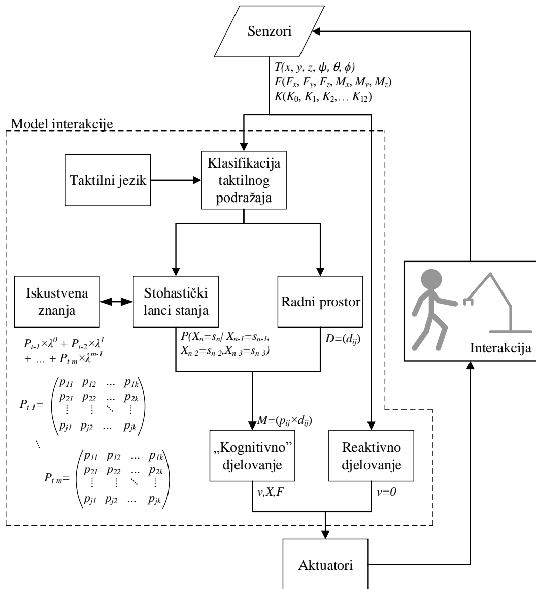
Slika 2.8. Predloženi model interakcije.
