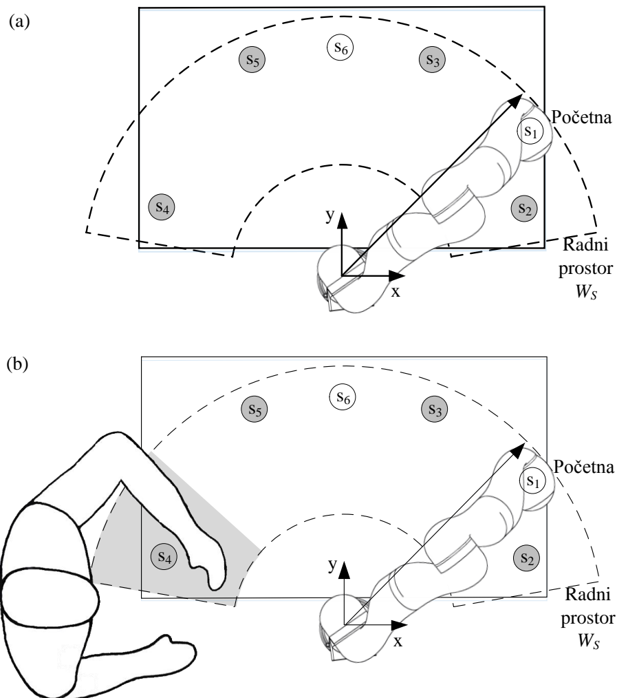
Slika 5.15. Radni prostor: a) slobodan, b) s čovjekom u radnom području.
