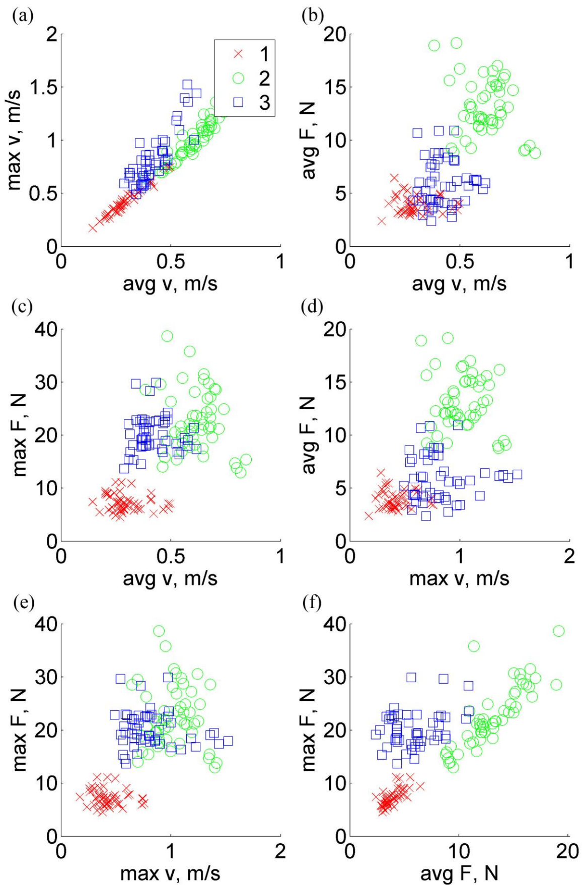
Slika 3.30. Dvokriterijski modeli klasifikacije.
