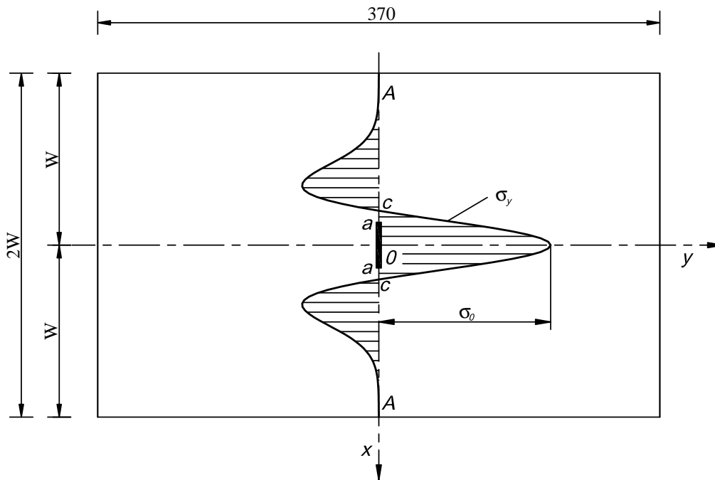
Slika 57. Sučeono zavarene ploče - analitički zadan profil zaostalih napreznaja
