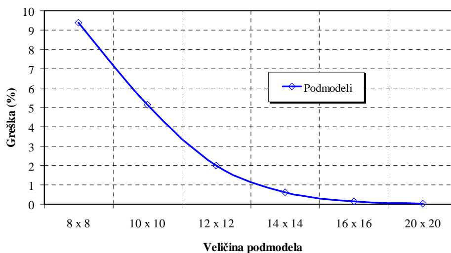
Slika 66. Utjecaj veličine podmodela na grešku koeficijenta intenzivnosti naprezanja kod sučeonog zavara dviju ploča
