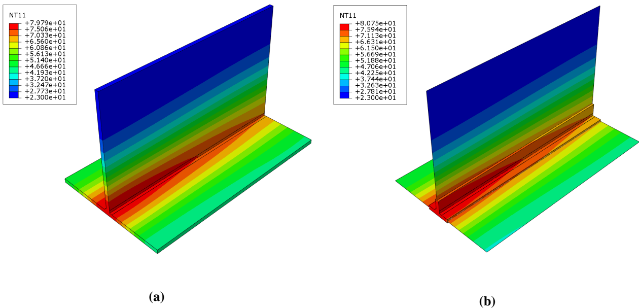
Slika 34. Raspodjela temperatura 290 s nakon početka zavarivanja: a) potpuni 3D model i b) kombinirani 3D/ljuskasti model
