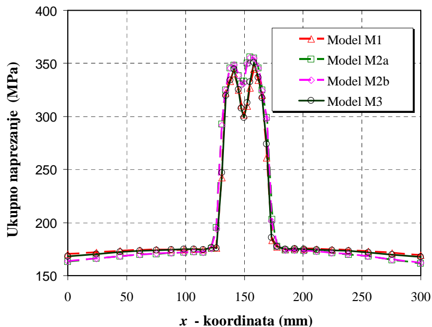
Slika 72. Profil ukupnih naprezanja u pravcu zavarivanja po srednjoj plohi horizontalne ploče (linija B-B, slika 20)
