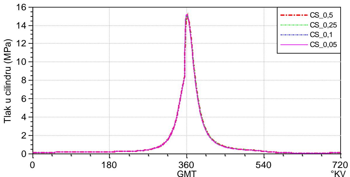
Slika 43. Verifikacija modela: utjecaj proračunskog koraka (0,5 do 0,05 °KV) na profil tlaka kod modela s 36 zona i konstanata SET 1
