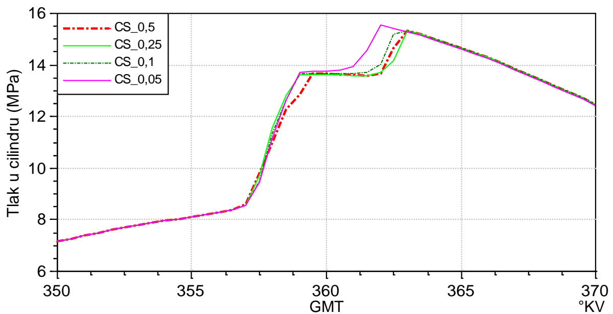
Slika 48. Verifikacija modela: utjecaj proračunskoga koraka (0,5 do 0,05 °KV) na profil tlaka kod modela s 12 zona i konstante SET 1 – uvećano u području GMT
