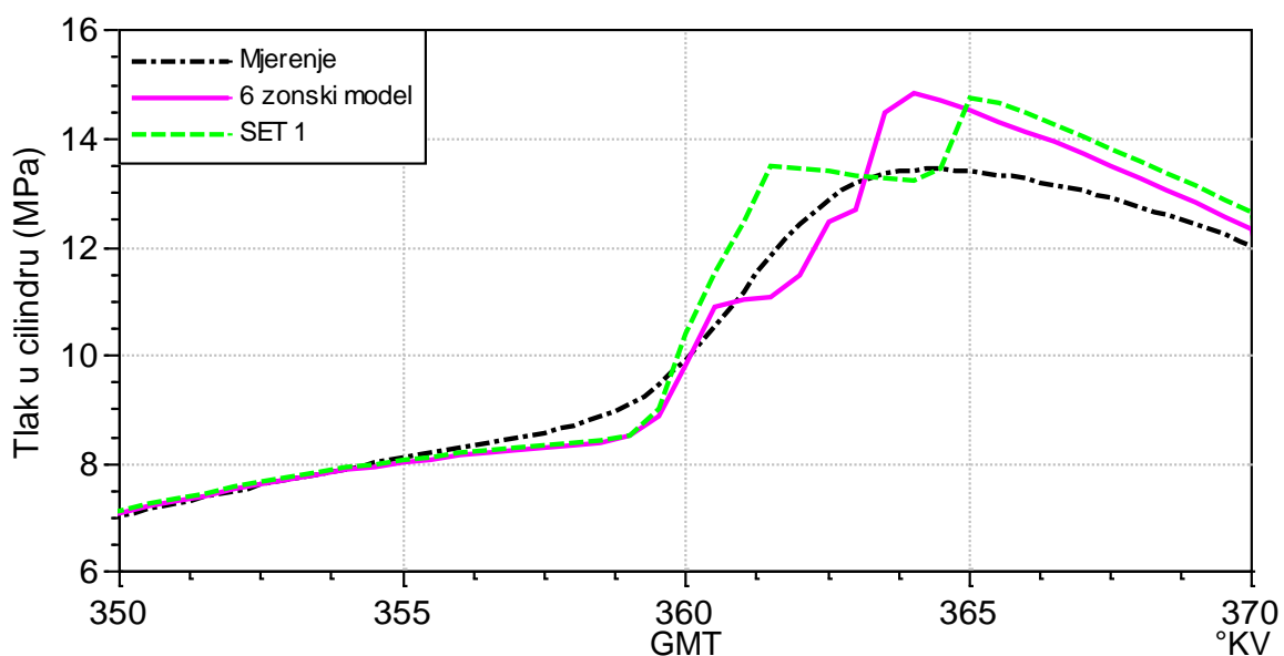
Slika 86. Validacija modela s 12 zona, SET 1: usporedba profila izmjenjenog tlaka i tlaka izračunatog simulacijskim modelima – uvećano u području GMT
