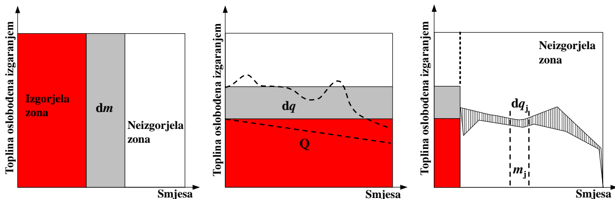
Slika 5. Prikaz oslobađanja topline Ottovog, HCCI i Dieselovog motora [11], [36]
