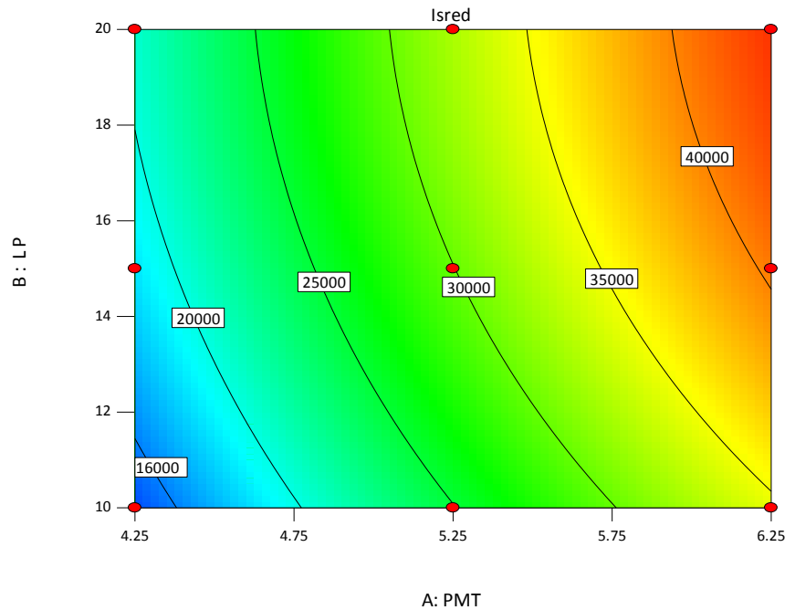
Sl.- 59. Konturni prikaz matematičkog modela ovisnosti odziva intenziteta zacrnjenja piksela digitalnog zapisa radiografske slike o parametrima očitavanja (konstantni su C:Res = 150 μm i D:EPS = 200 kPa).
