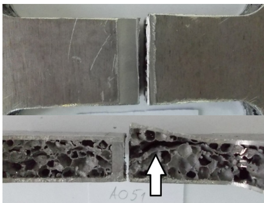
Slika 6.29. Prijelom epruvete A051
