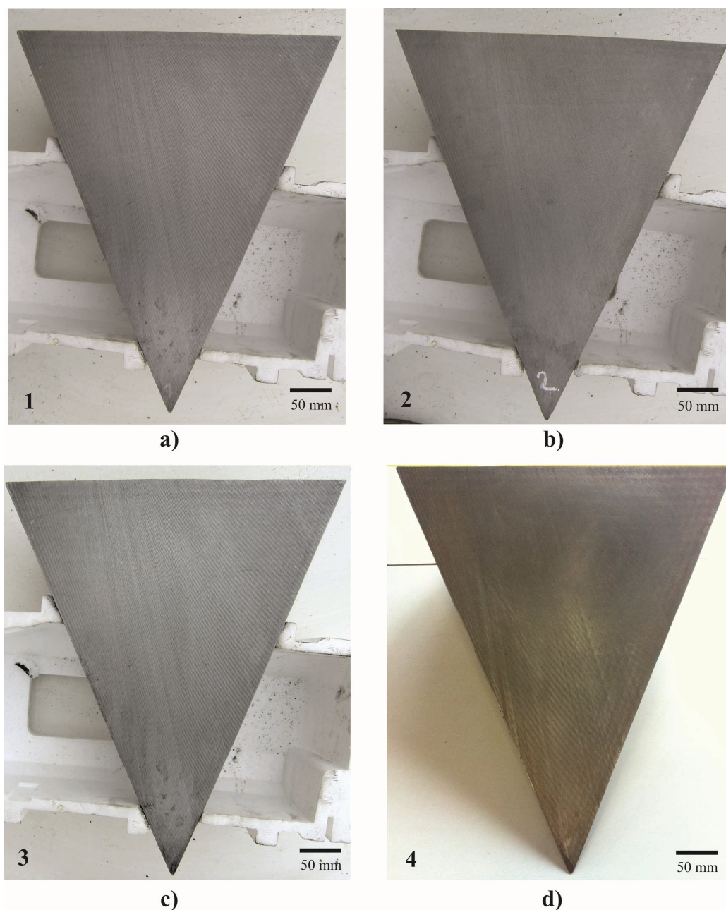
Slika 4.12 Makroslike poprečnih presjeka stožaca 1 do 4 (EN-GJS-400-15): a) cijepljenje u lonac, b) cijepljenje u lonac + 0,01 % Bi, c) cijepljenje u mlaz, d) cijepljenje u mlaz + 0,01 % Bi
