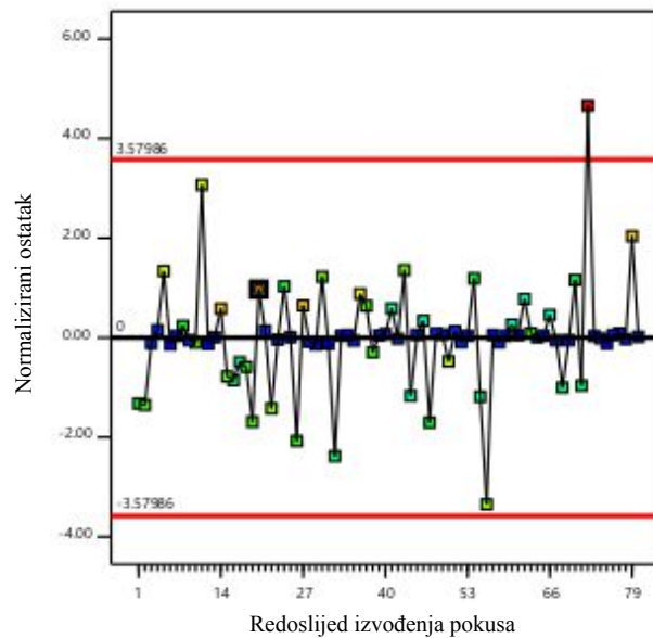
Slika 40. Slučajno rasipanje ostataka u odnosu na redosljed izvođenja plana za matematički model za izračun vodećeg vremena kod upravljanja procesom hibridnim mehanizmom upravljanja
