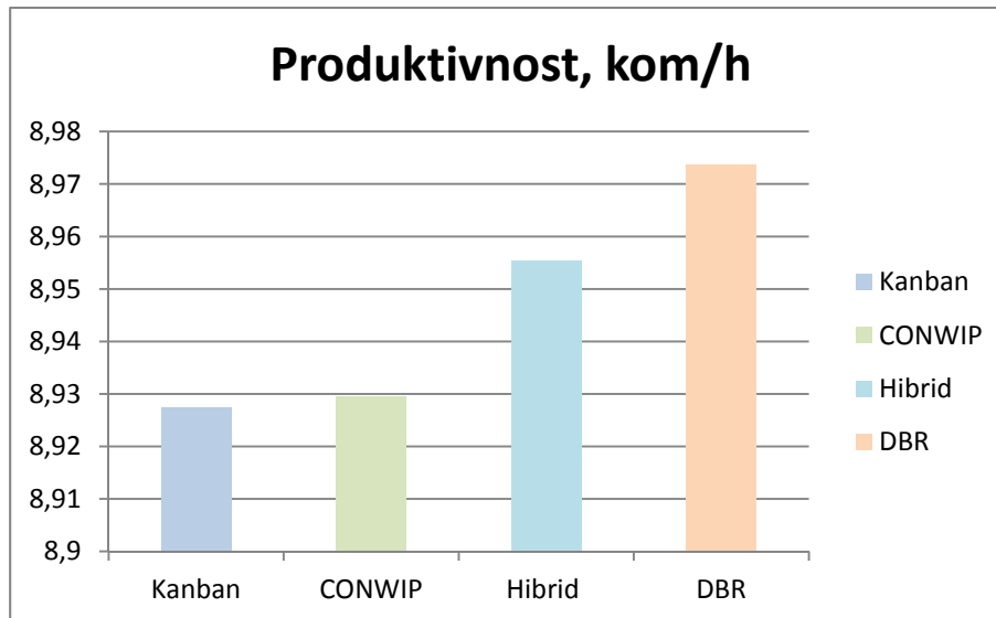
Slika 60. Usporedba mjerne performanse produktivnost za C_v=0,25 , t=5 min za proces koji ima usko grlo, WIP=15
