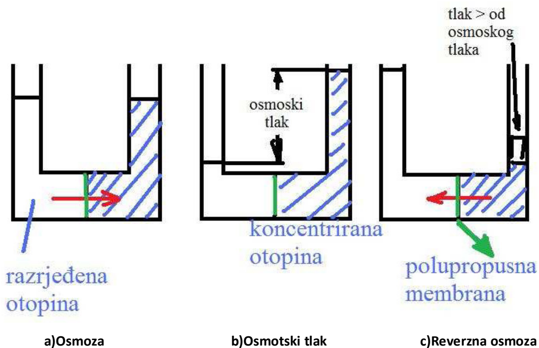
Slika 6. Schematski prikaz osmoze i reverzne osmoze
