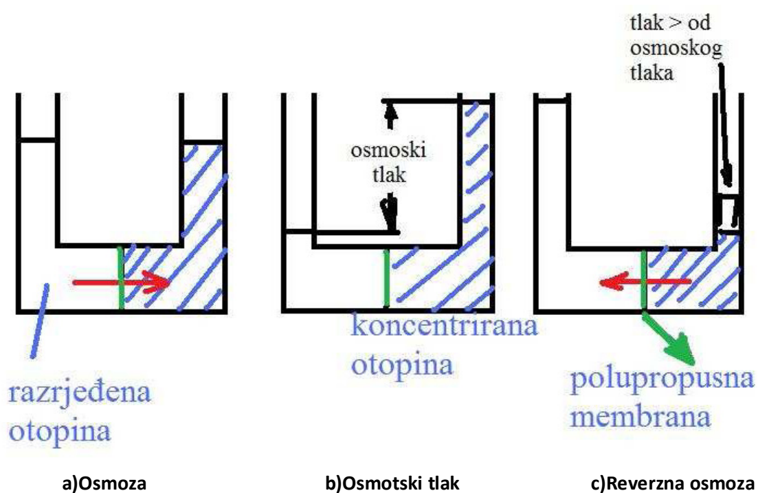
Slika 6. Shematski prikaz osmoze i reverzne osmoze
