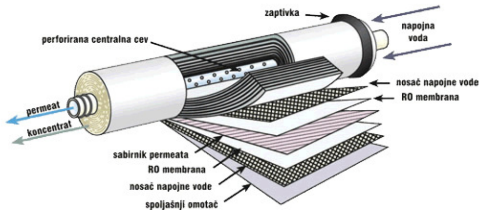
Slika 8. Presjek modula
