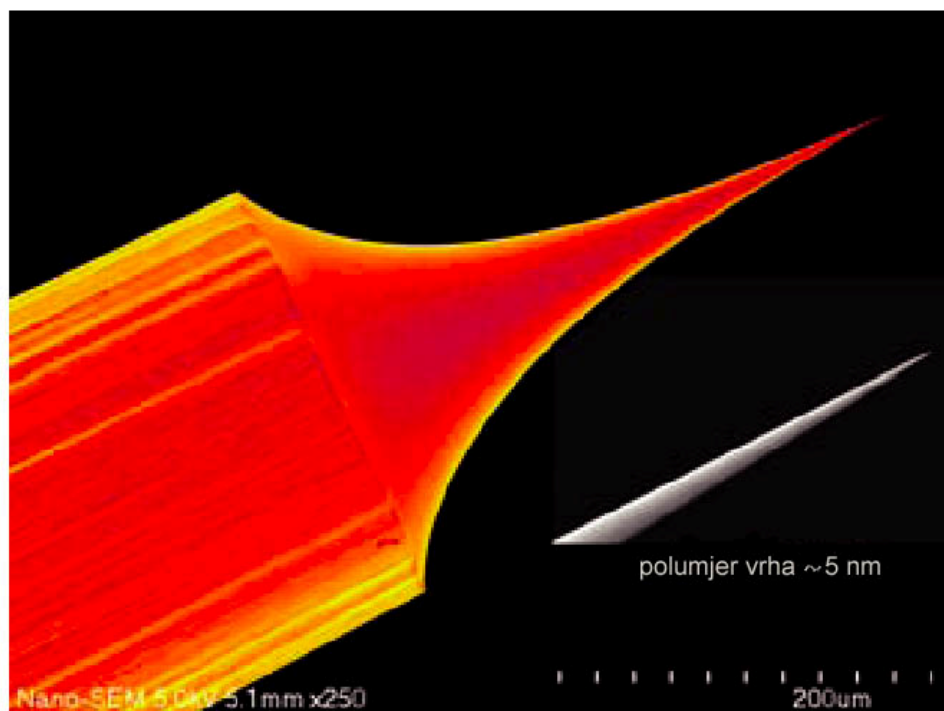
Slika 19. Volframski nano-vrh [1]
