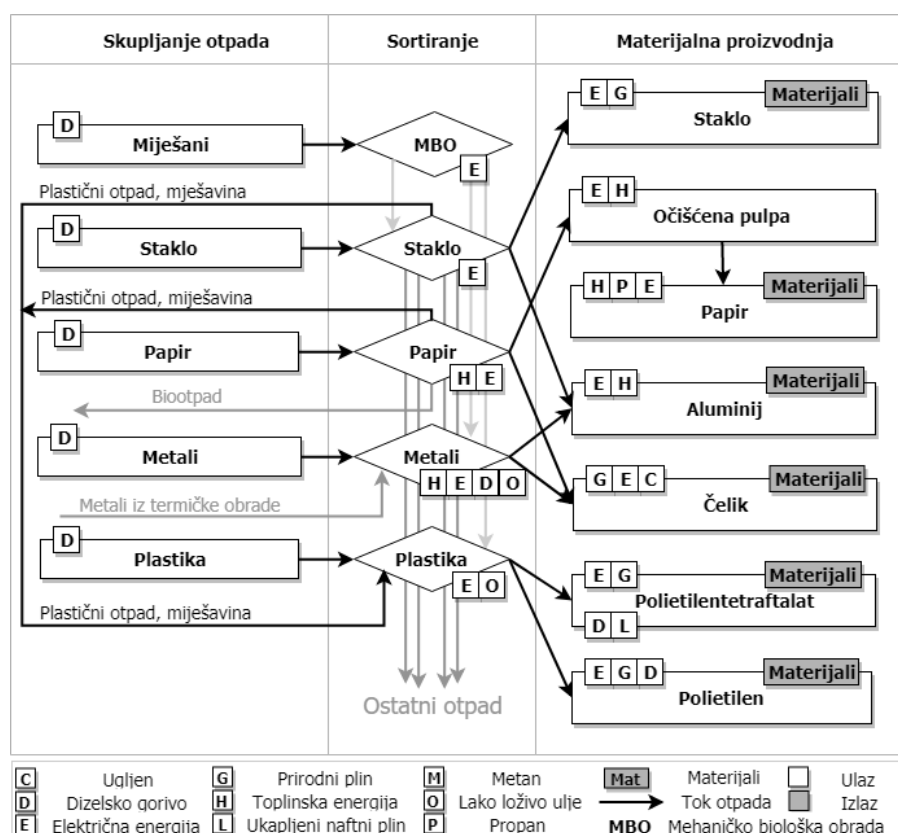
Slika 10. Tehnologije sortiranja otpada te primjer njihovog povezivanja u sustav
