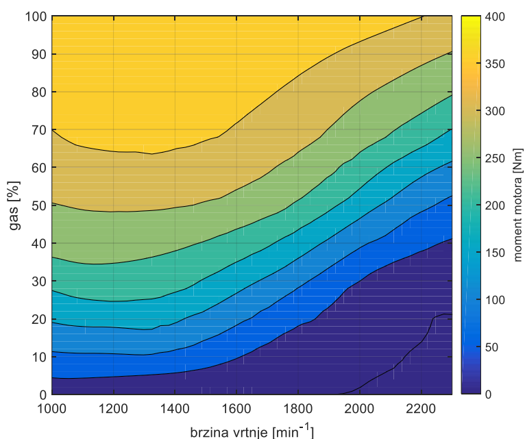
Slika 10. Mapa ovisnosti momenta motora o brzini vrtnje i papučici gasa
