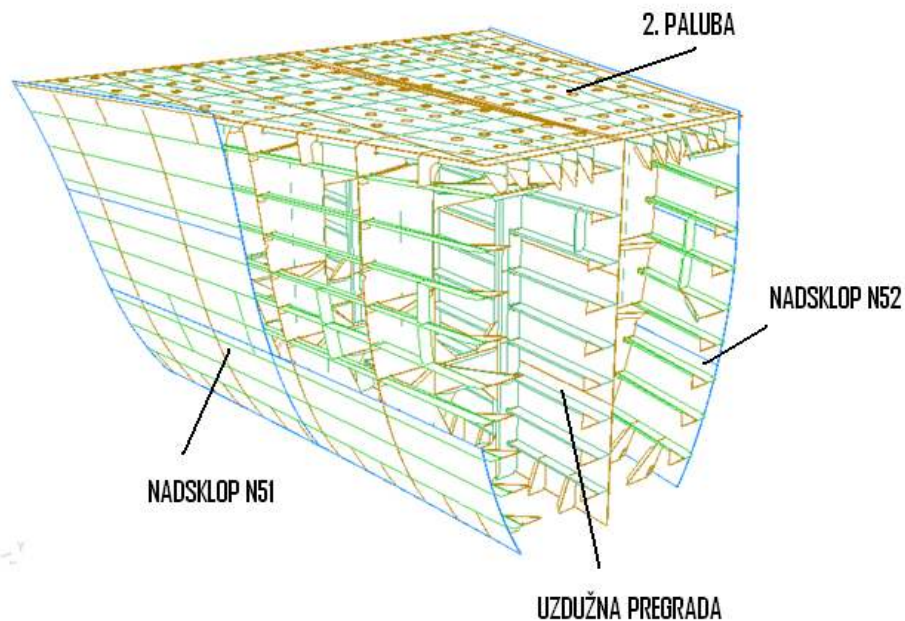
Slika 48. Izometrijski prikaz sekcije 3251
