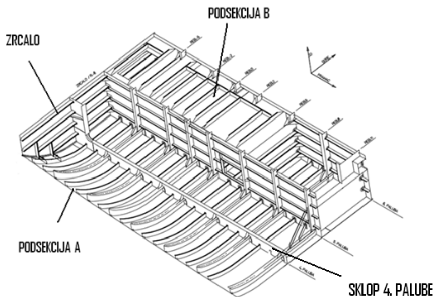
Slika 38. Izometrijski prikaz sekcije 3381
