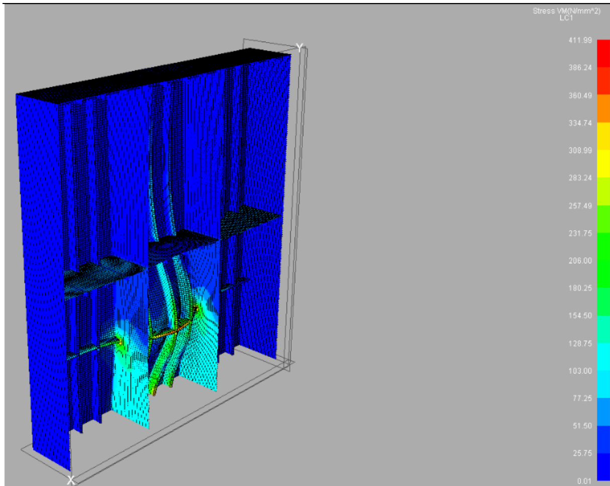
Slika 28. Ekvivalentna naprezanja redimencioniranog modela za prvi slučaj opterećenja
