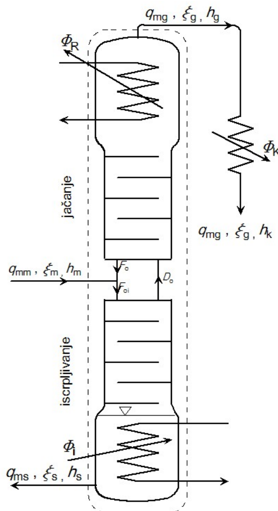
Slika 7. Spojena kolona [5]
