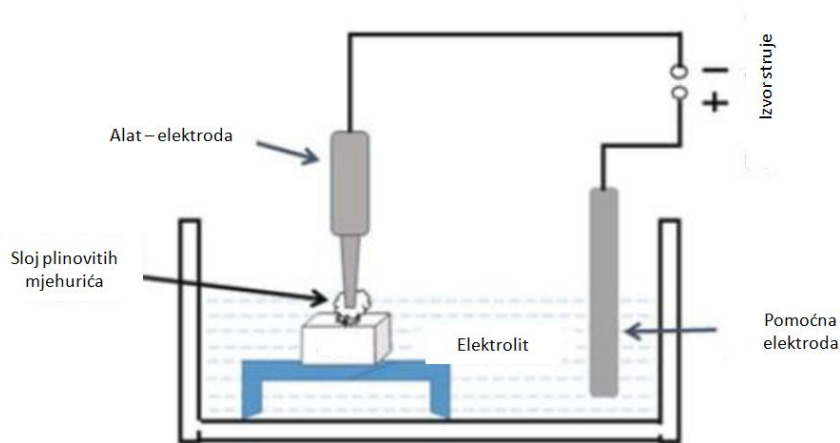
Slika 56. Shematski prikaz EDCM postupka [50]
