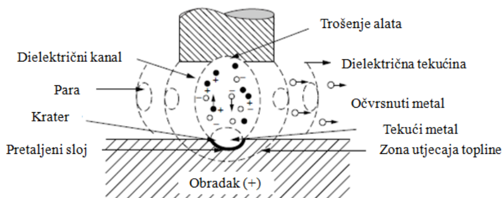
Slika 20. Električno pražnjenje [3]
