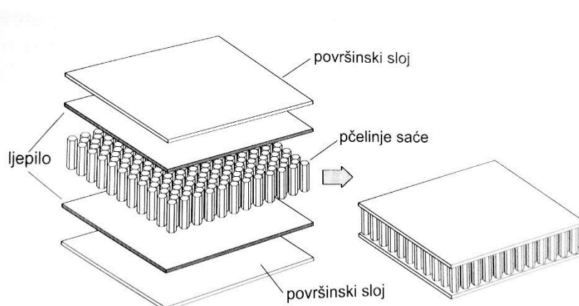
Slika 4. Primjer sendvič konstrukcije [3]
