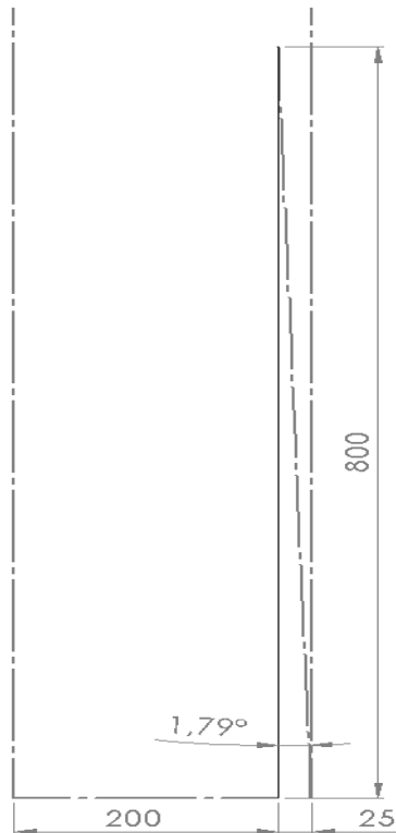
Slika 42. Kut između vlakna i izvodnice spremnika
