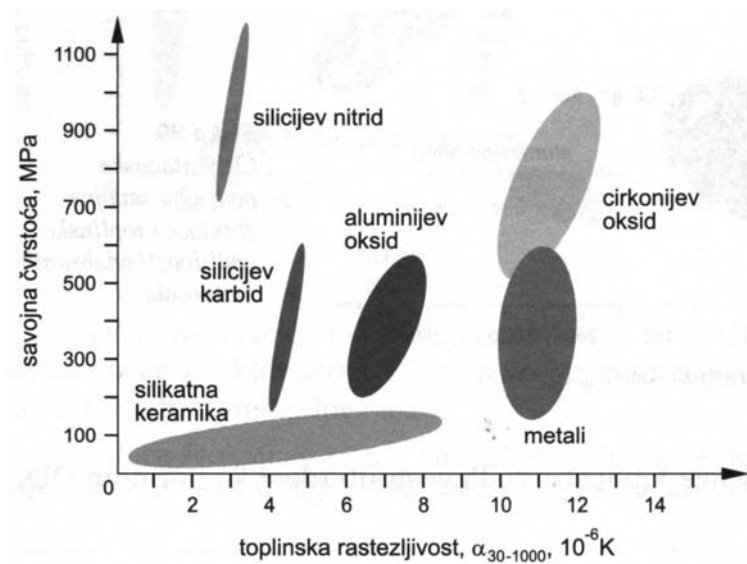
Slika 17 Orijetacijska područja savojne čvrstoće i toplinske rastezljivosti [1]
