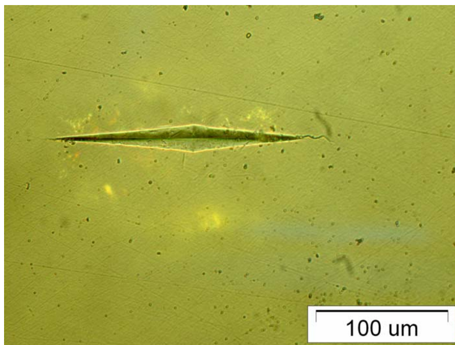
Slika 39 Otisak dijamentne piramide nakon mjerenja tvrdoće metodom HK5
