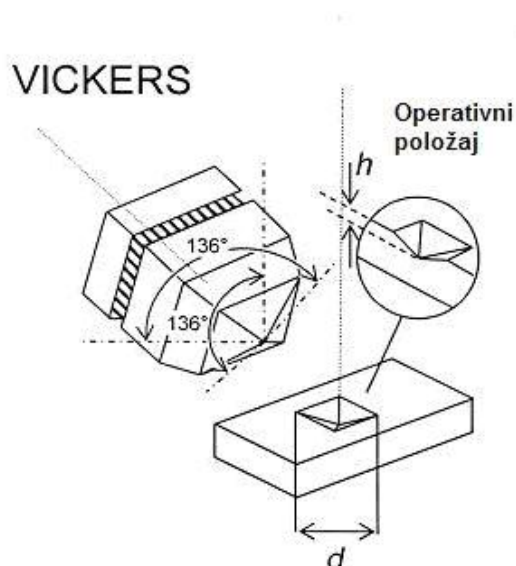
Slika 20 Shematski prikaz Vickersovog penetratora i otiska [11]
