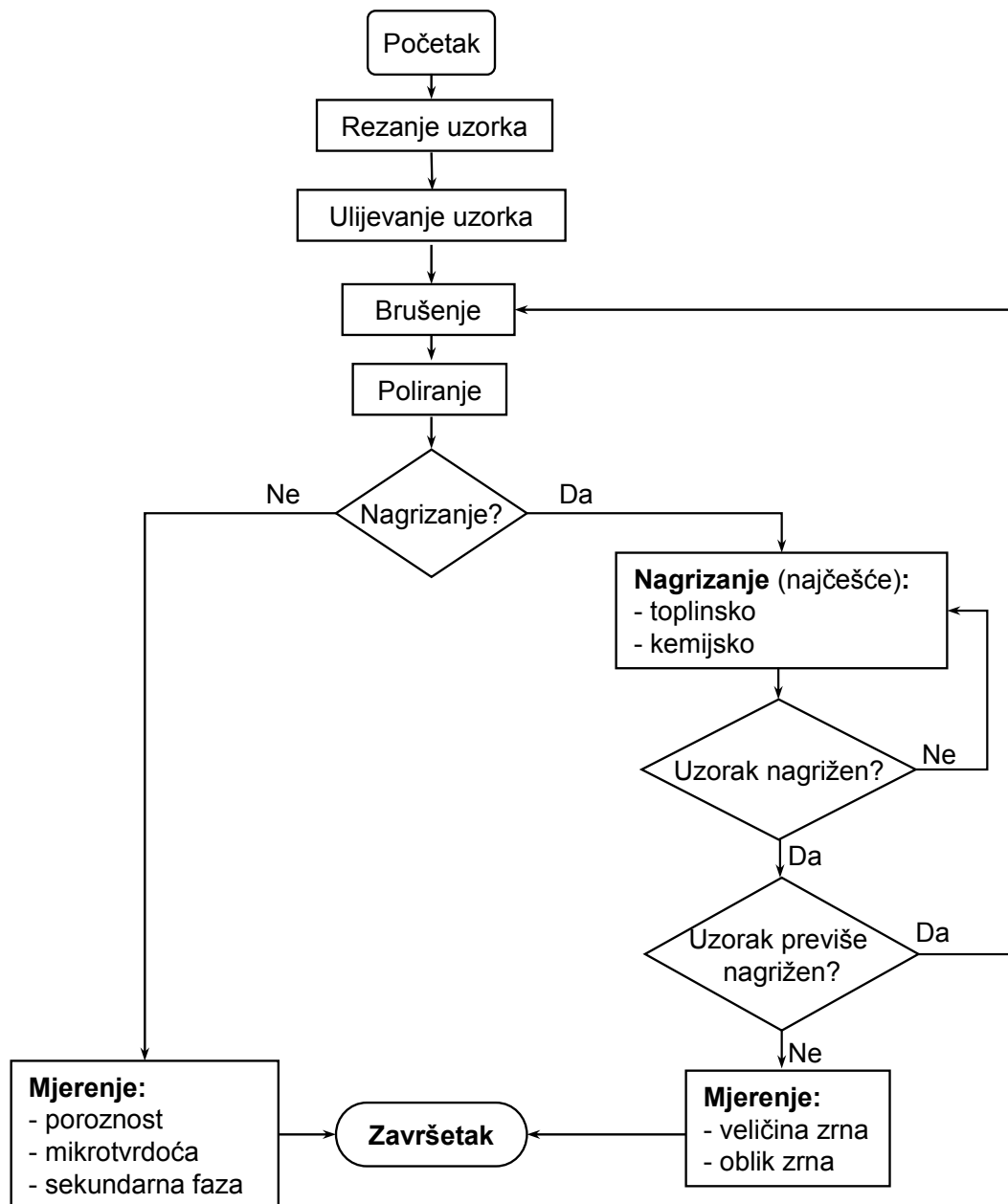
Slika 18 Dijagram tijeka pripreve uzorka za keramografiju [9]
