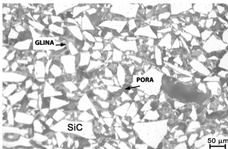
Slika 2 Mikrostruktura sitnozrnatog silicijeva karbida povezanog silikatima [1]
