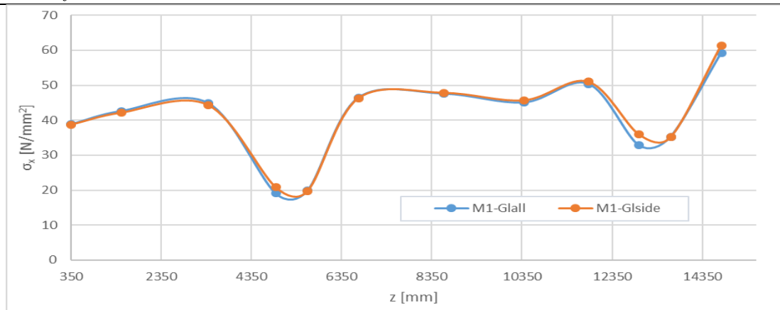
Slika 33 Raspodjela \sigma_x napreznja modela M1 po širini palube šest
