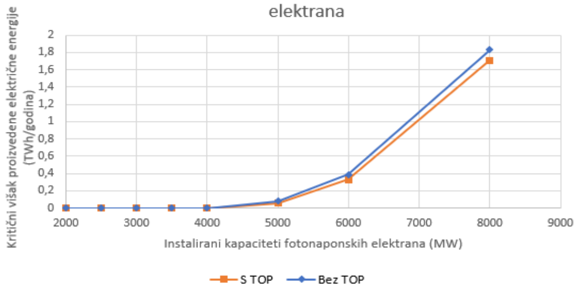
Slika 20. Krivulje promjene kritičnog viška proizvedene električne energije promjenom instaliranih kapaciteta fotonaponskih elektrana
