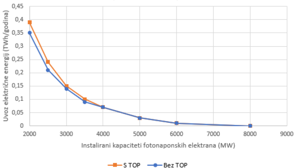
Slika 22. Krivulje promjene uvoza električne energije promjenom instaliranih kapaciteta fotonaponskih elektrana
