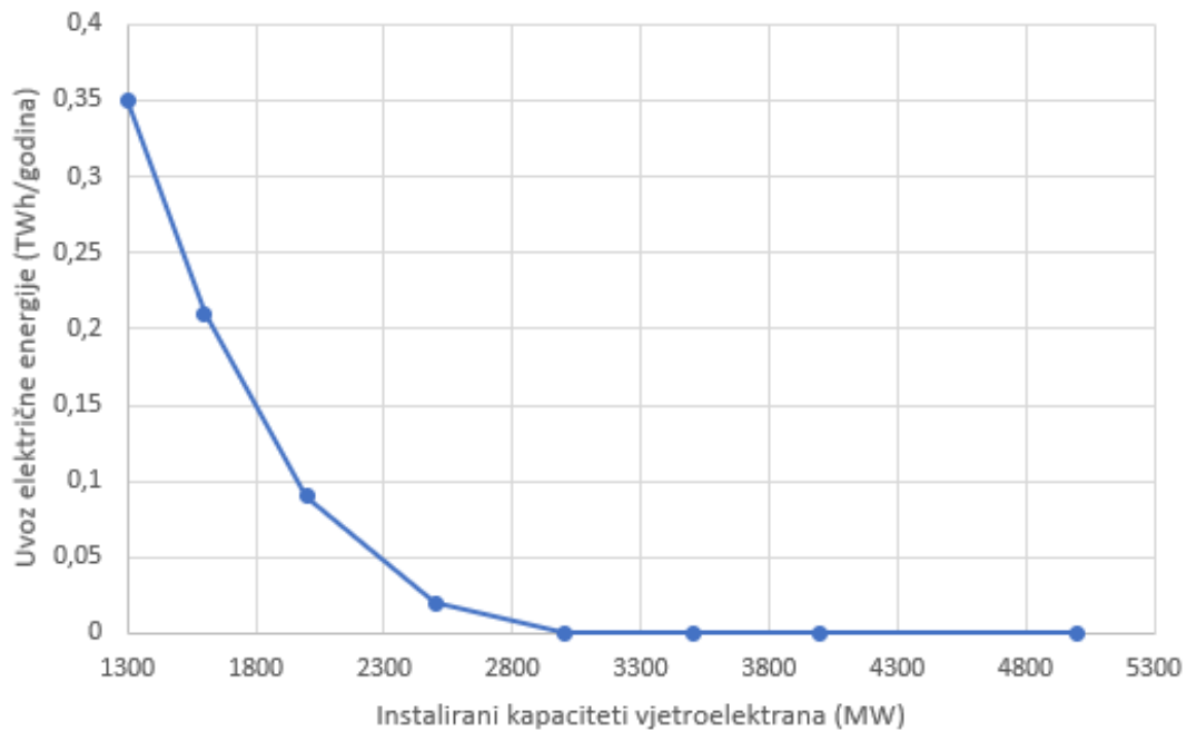
Slika 15. Krivulja promjene uvoza električne energije promjenom instaliranih kapaciteta vjetroelektrana
