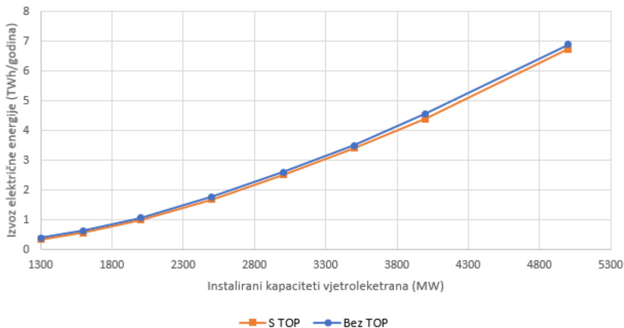
Slika 27. Krivulje promjene izvoza električne energije promjenom instaliranih kapaciteta vjetroelektrana
