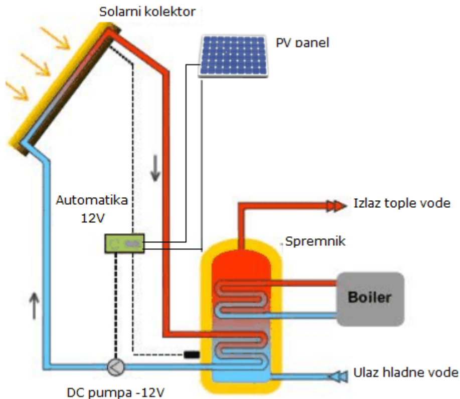
Slika 1. Shema solarnog toplinskog sustava [6]
