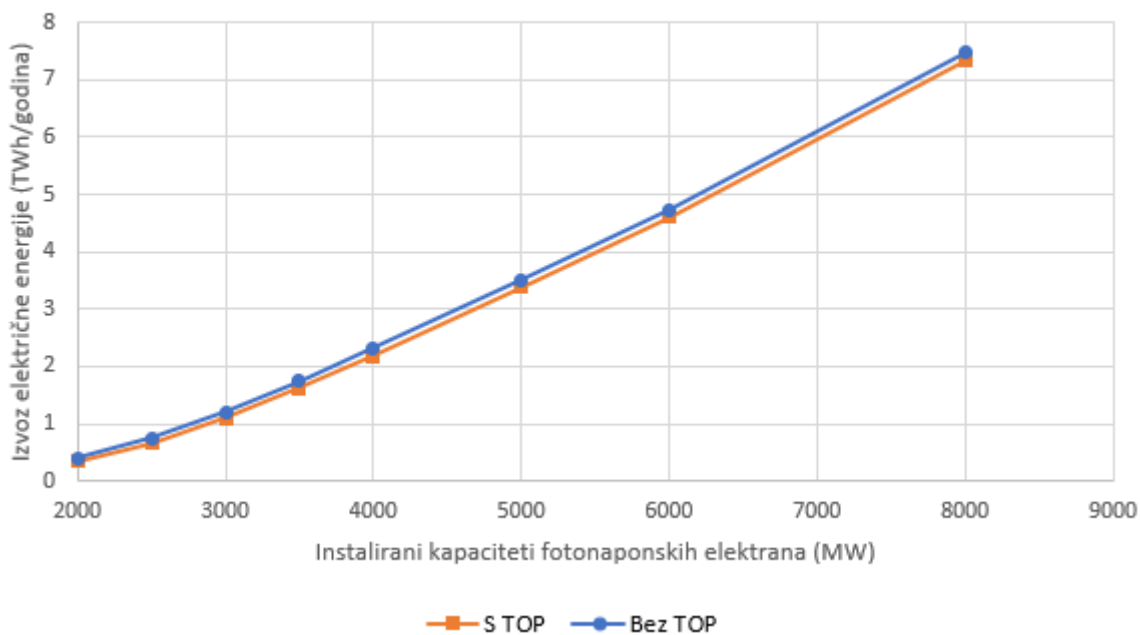
Slika 23. Krivulje promjene izvoza električne energije promjenom instaliranih kapaciteta fotonaponskih elektrana
