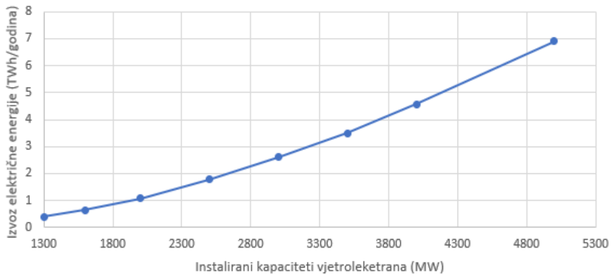
Slika 16. Krivulja promjene izvoza električne energije promjenom instaliranih kapaciteta vjetroelektrana
