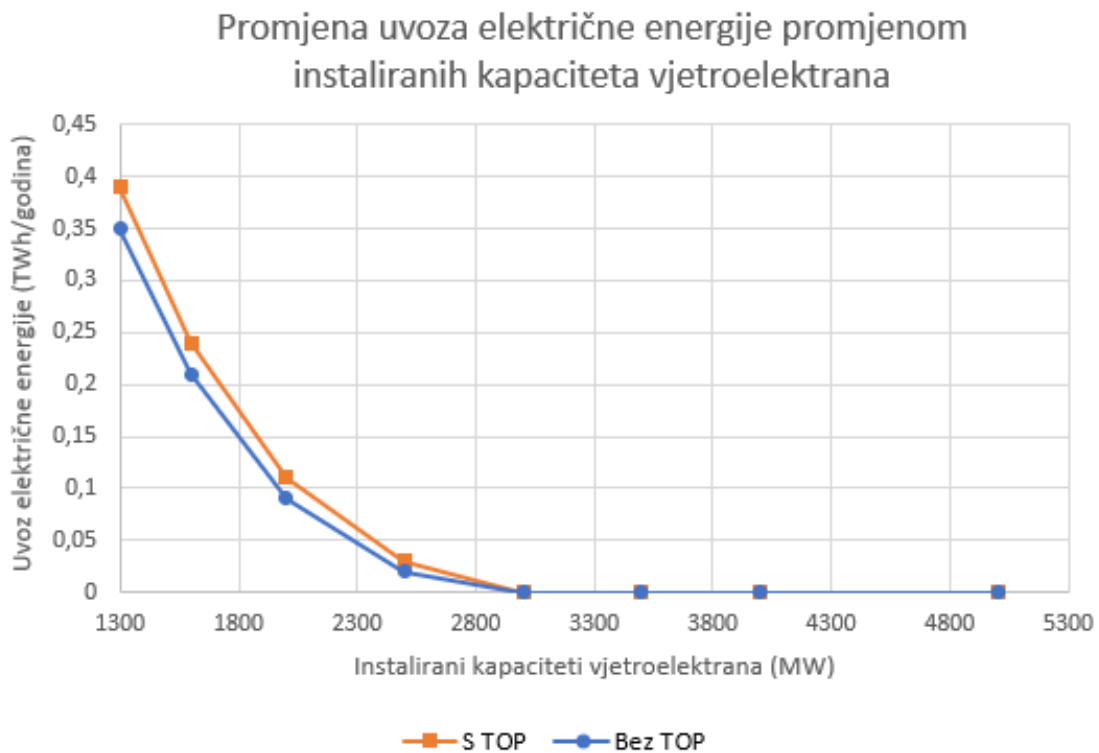
Slika 26. Krivulje promjene uvoza električne energije promjenom instaliranih kapaciteta vjetroelektrana
