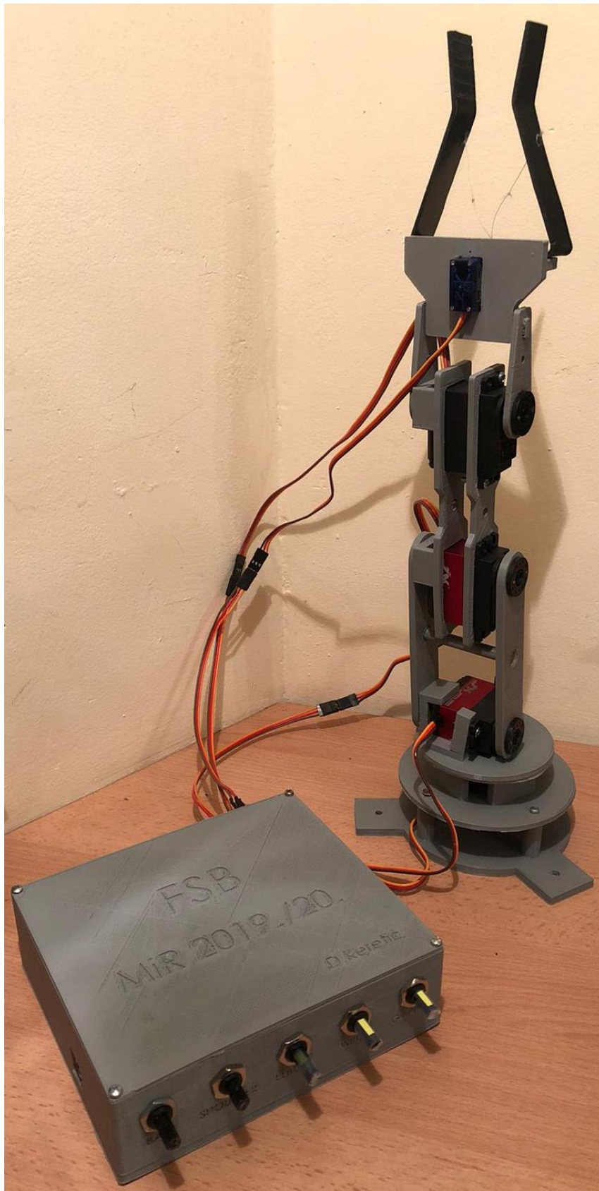
Slika 44. Završni sklop
