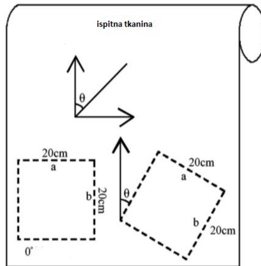
Slika 1.8. Ispitni uzorci [14]
