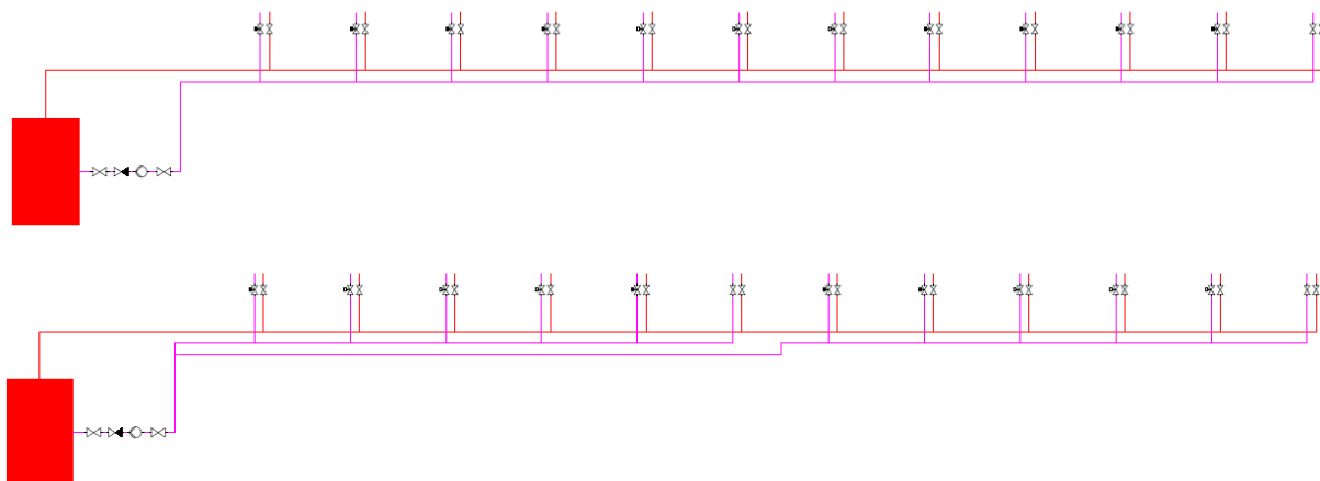
Slika 20. Poboljšanje hidrauličkih uvjeta paralelnim postavljanjem glavnog razvoda, izrađeno prema [20]
