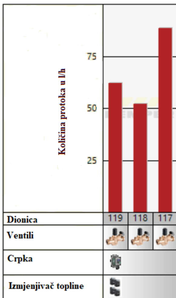
Slika 29. Zagrijavanje vode: Sustav za pripremu tople vode – temperatura: 60 °C
