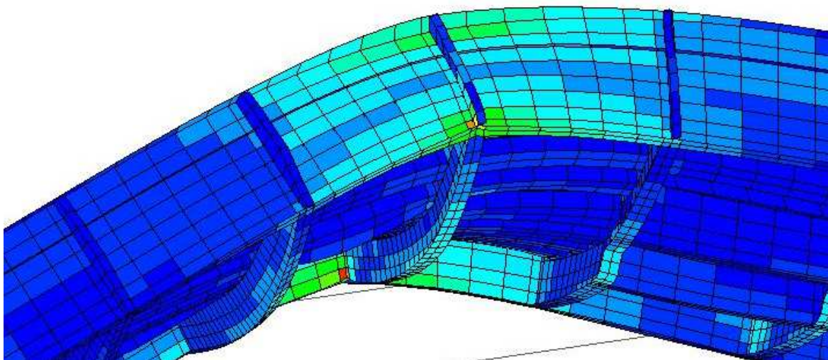
Slika 24. Najveća von Mises naprežanja
