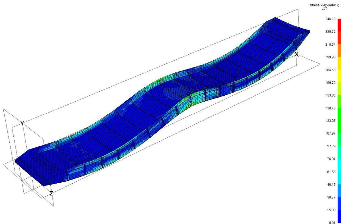
Slika 28. Naprezanja von Mises LCH-2
