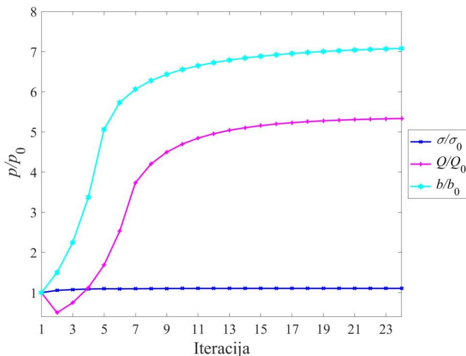
Slika 33. Prikaz promjene parametara izotropnog očvršćenja po iteracijama kod jednoosnog monotono opterećenja
