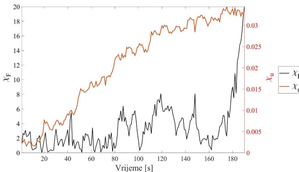
Slika 27. Razlika funkcionala \chi_F i \chi_u u zadnjoj iteraciji identifikacije modula elastičnosti kod jednoosnog monotonomog opterećenja
