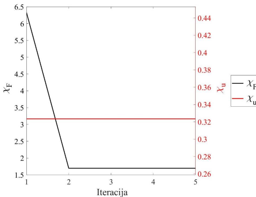
Slika 26. Vrijednosti funkcionala \chi_F i \chi_u po iteracijama identifikacije modula elastičnosti kod jednoosnog monotonomog opterećenja
