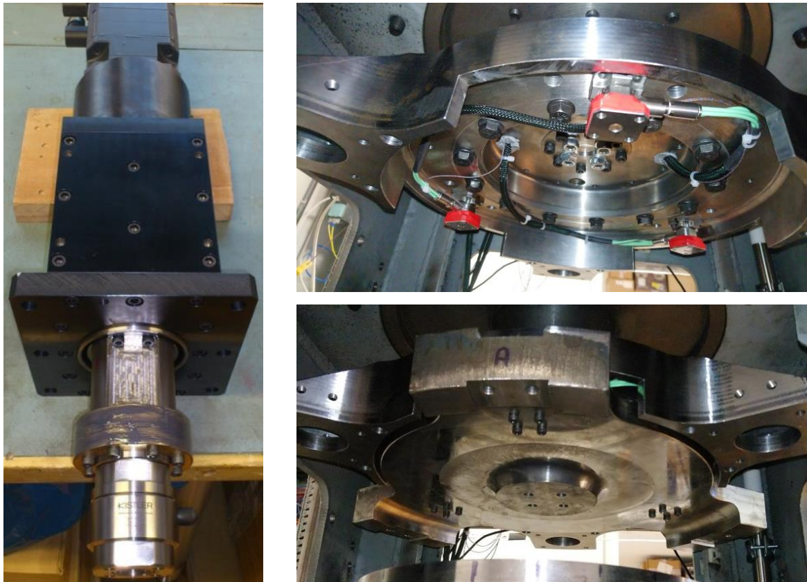
Slika 43. Vertikalna os s inicijalnom izvedbom (lijevo) i s tri troosna senzora (desno) ([32])
