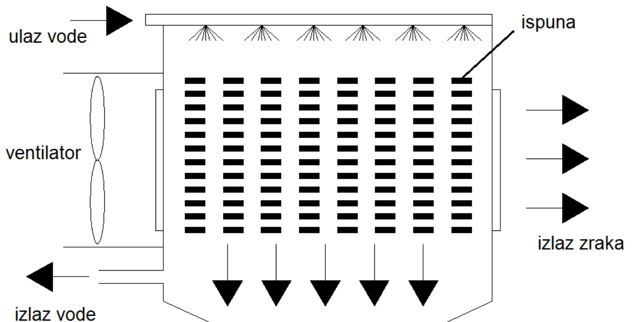
Slika 10. Križno strujanje
