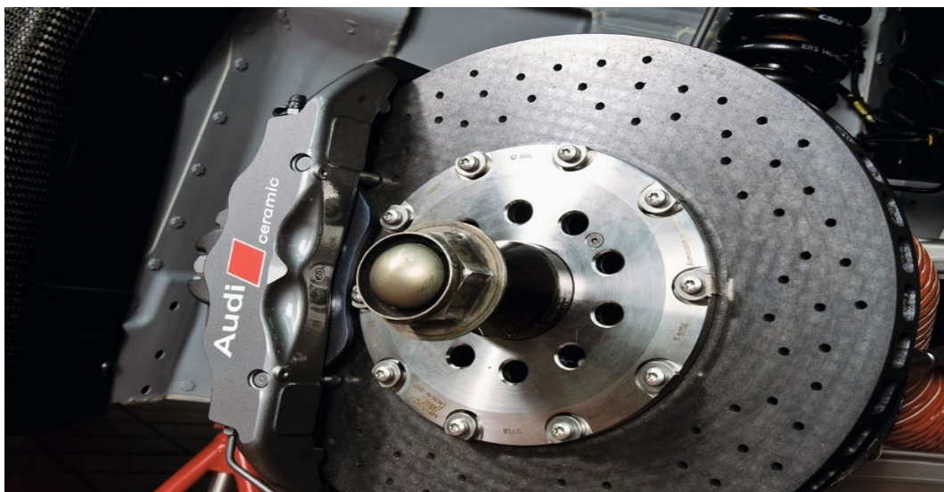
Slika 2. Keramičke disk-kočnice [3]
