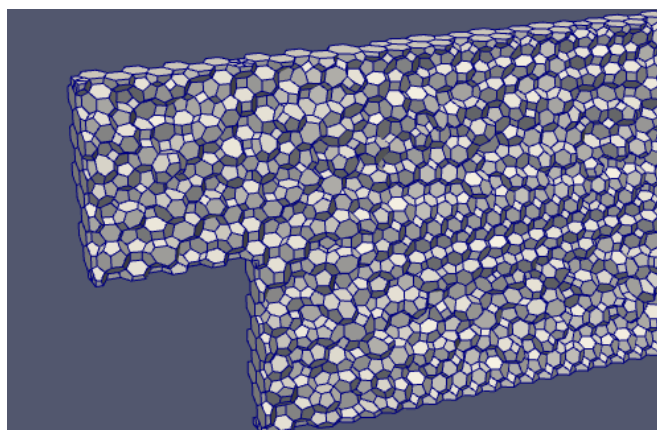
Slika 5.12. Poliedarska mreža
