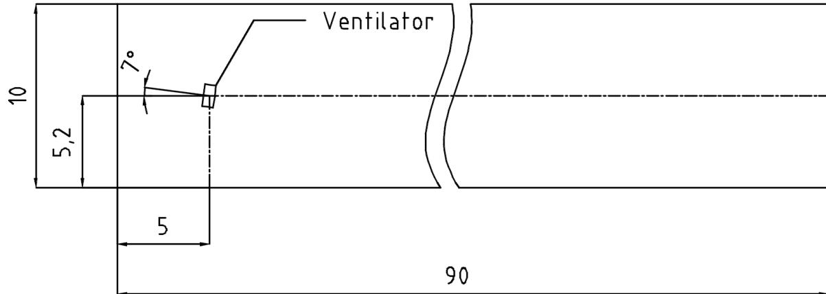
Slika 5.2. Geometrijski model
