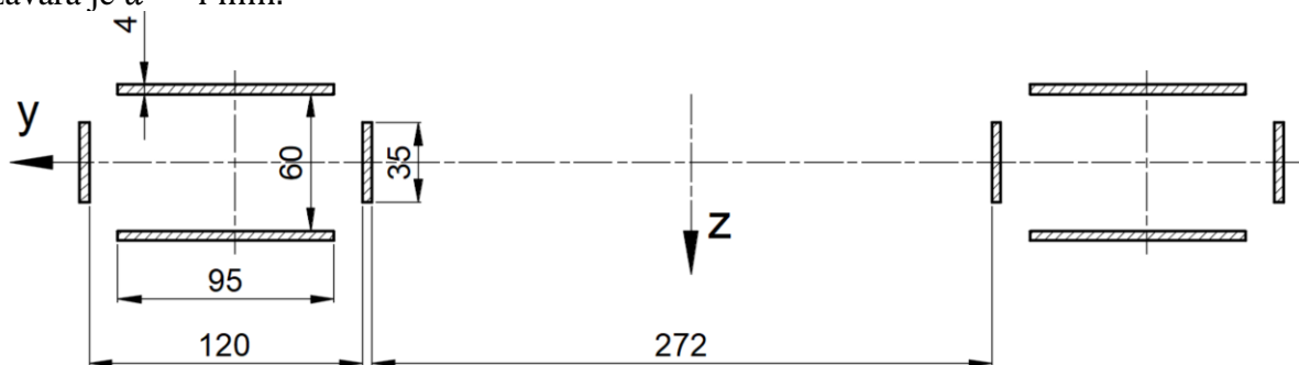
Slika 6.27. Poprečni presjek zavora nosive konstrukcije
