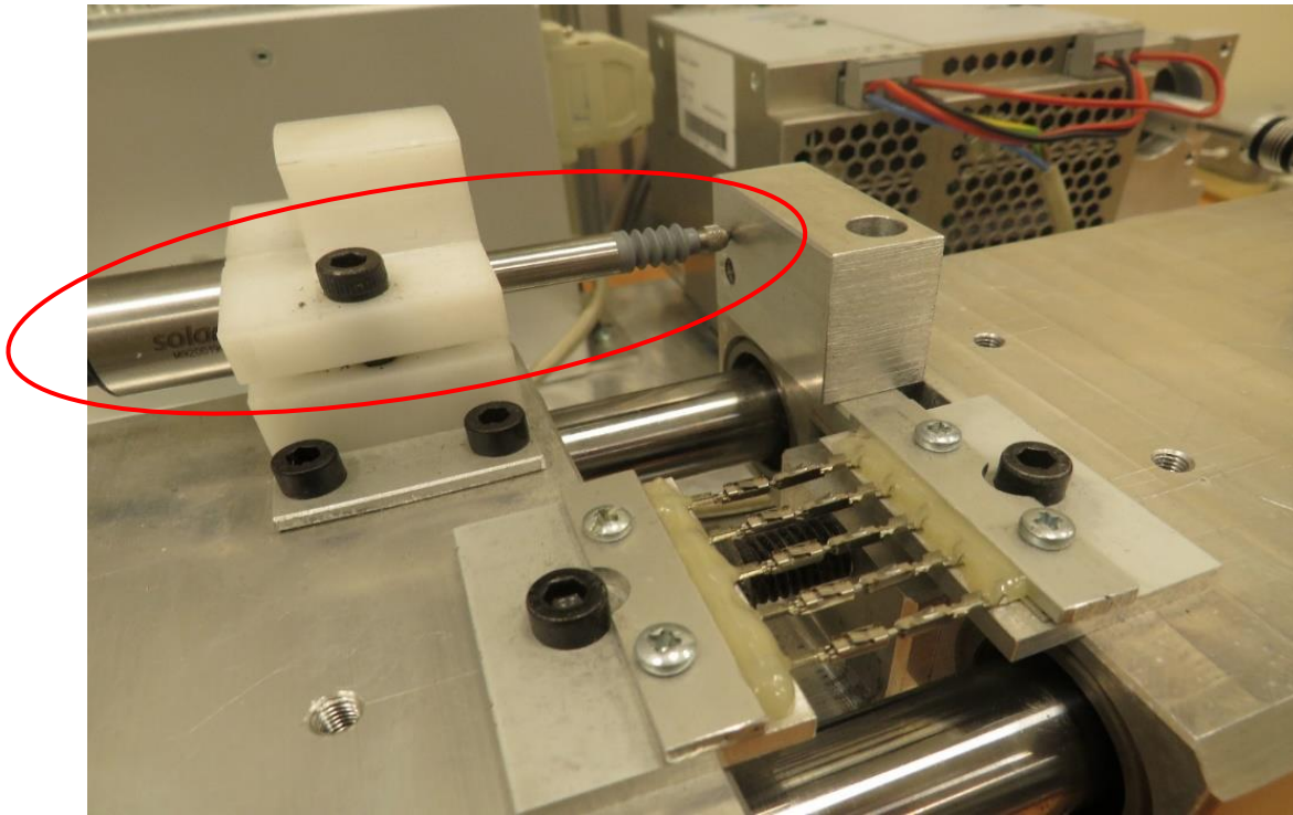
Slika 24. Senzor pomaka
